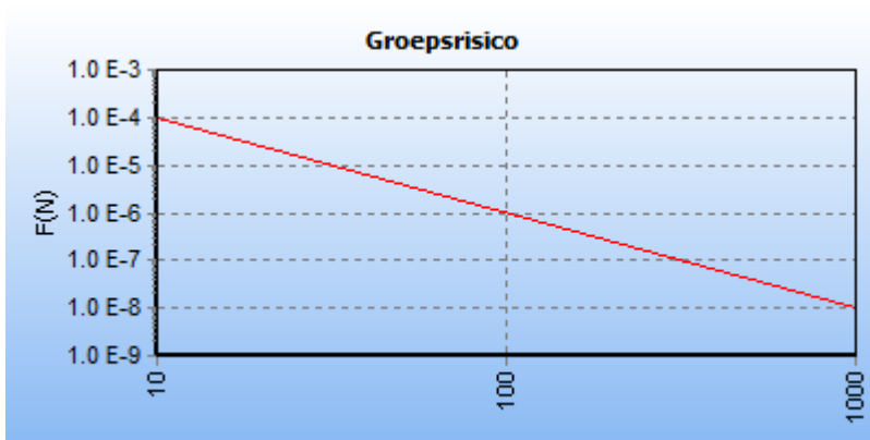
Figuur 10: fN-curve van de kilometer met de hoogste overschrijdingsfactor van gastransportleiding N-524-08 in de toekomstige situatie.
