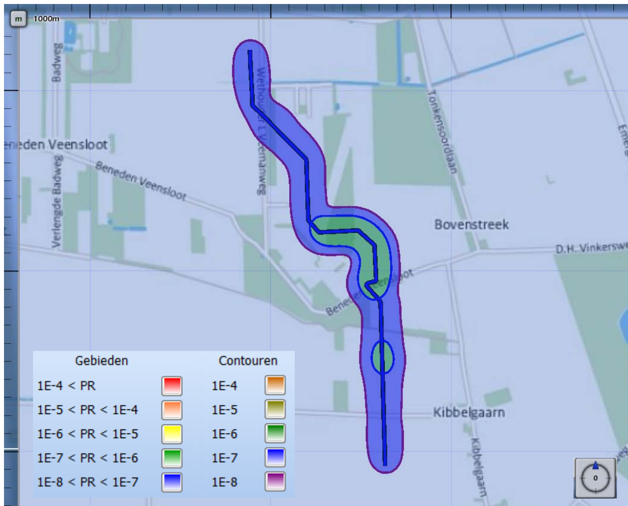
Figuur 6: PR van gastransportleiding N-524-08 toekomstige situatie.
