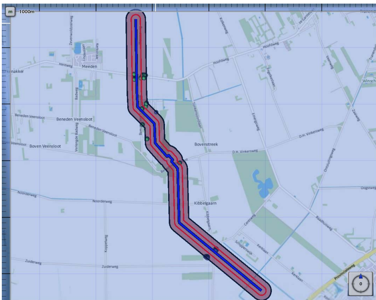
Figuur 3: Bevolkingsgegevens rondom de leiding N-524-08 excl. verlegging zoals aangeleverd door de BAG populatieservice.
