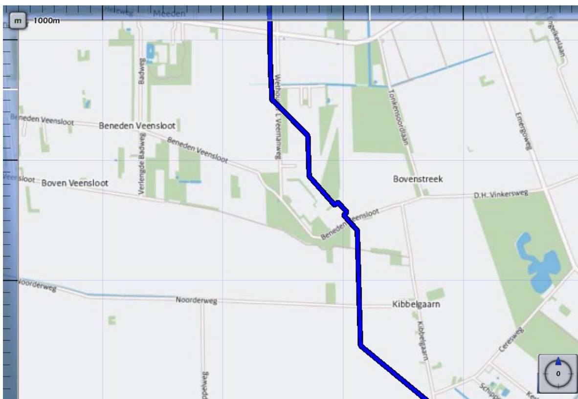
Figuur 1: Ligging van gastransportleidingen N-524-08 huidige situatie.
