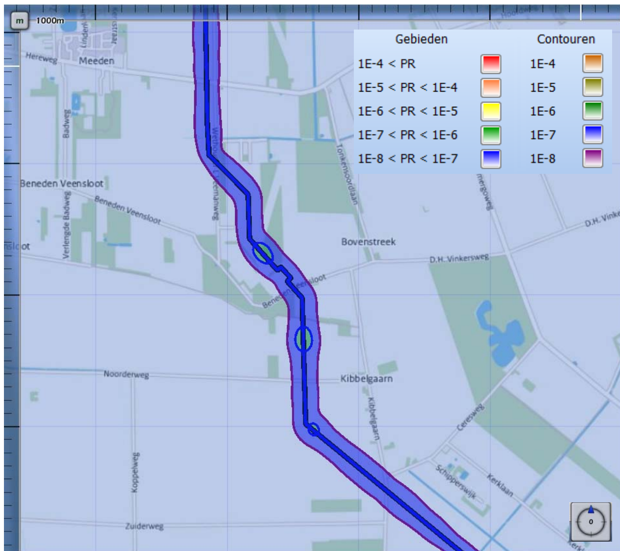
Figuur 5: PR van gastransportleiding N-524-08 huidige situatie.
