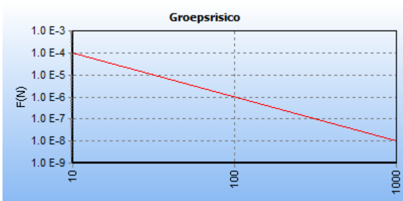
Figuur 8: fN-curve van de kilometer met de hoogste overschrijdingsfactor van gastransportleiding N-524-08 in de huidige situatie.
