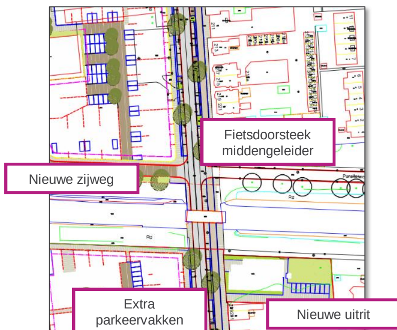
Figuur 6.1 Infrastructurele aanpassingen in nabijheid spoorwegovergang
