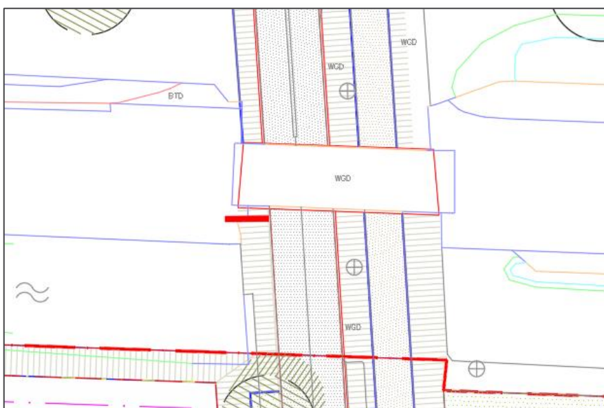
Figuur 7.4 Overwegboom trottoir voor spoorwegovergang
