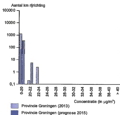
Concentratiehistogram PM 10
