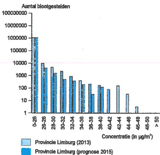
Blootstellingshistogram NO 2
