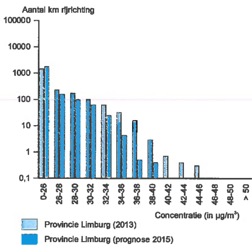
Concentratiehistogram NO 2
