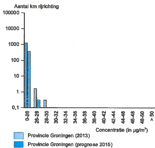
Concentratiehistogram NO 2
