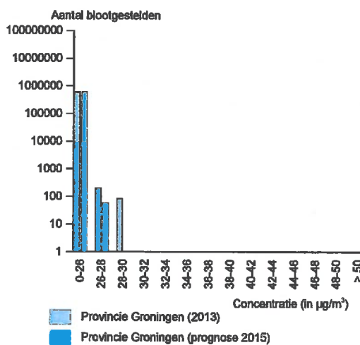
Blootstellingshistogram NO 2
