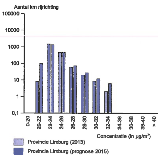
Concentratiehistogram PM 10
