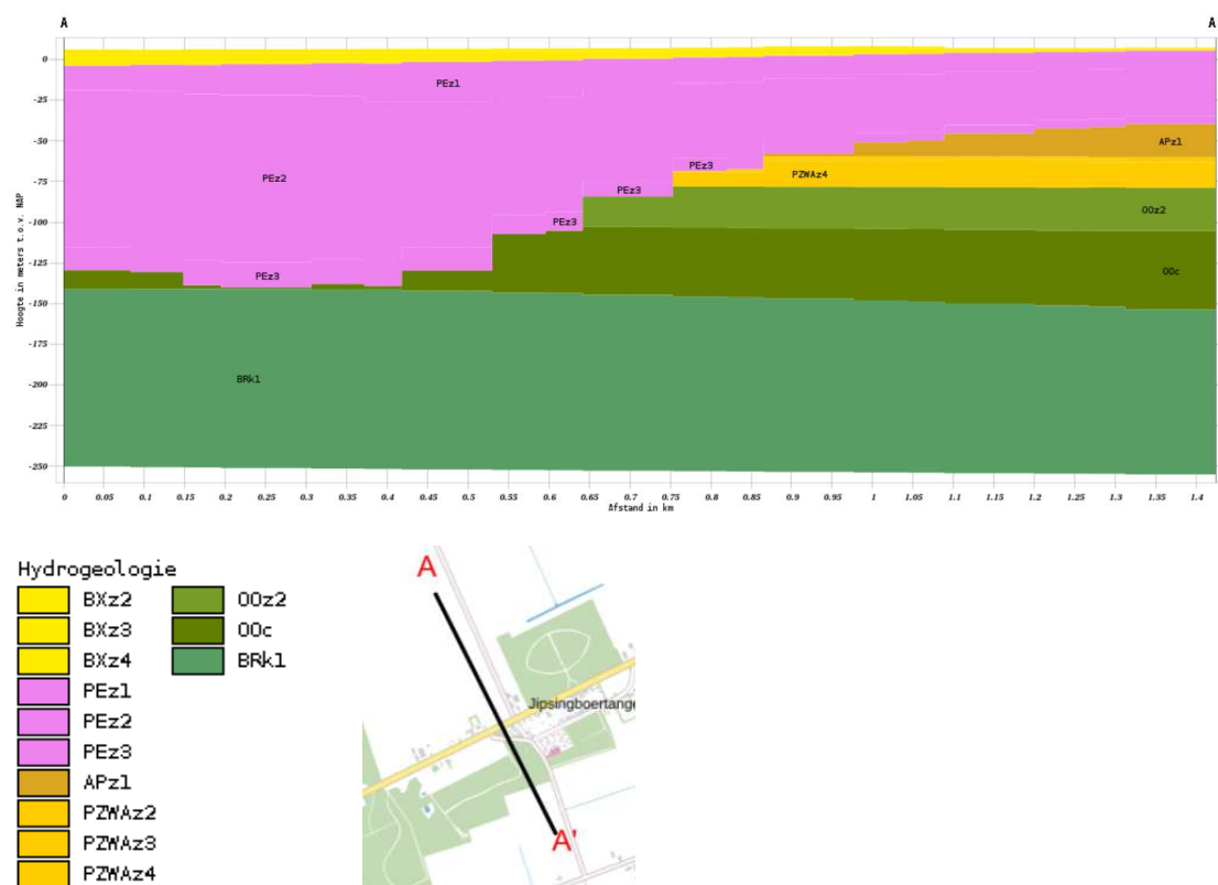
figuur 2: geohydrologische opbouw
