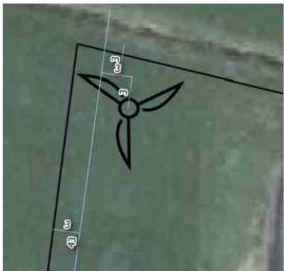
detail positie turbine t.o.v. bouwblokgrens en insteek sloot
