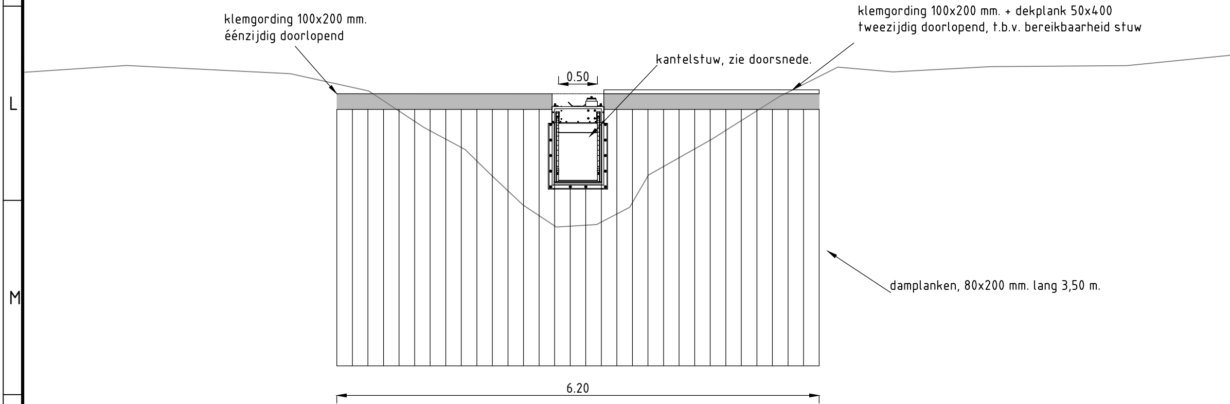
Kantelstuw Schaal 1:50
