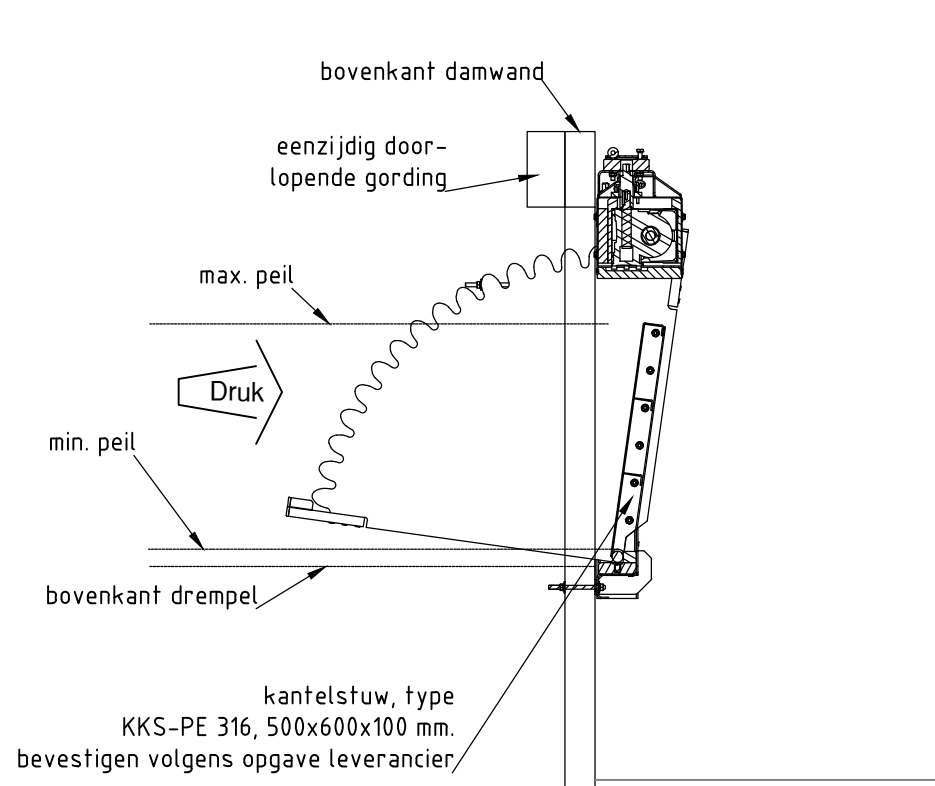
Doorsnede kantelstuw Schaal 1:20
