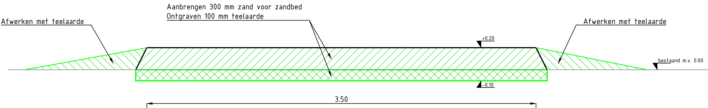
Principeprofiel herstellen zandpad Schaal 1:20
