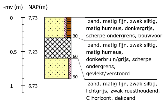
Boring 42 RD-coördinaten: 266205/550027
