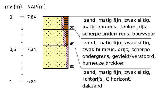
Boring 26 RD-coördinaten: 266006/550203
