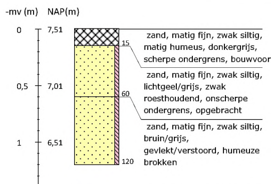
Boring 82 RD-coördinaten: 266026/550444
