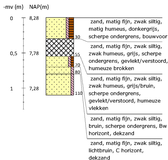
Boring 51 RD-coördinaten: 266286/550225
