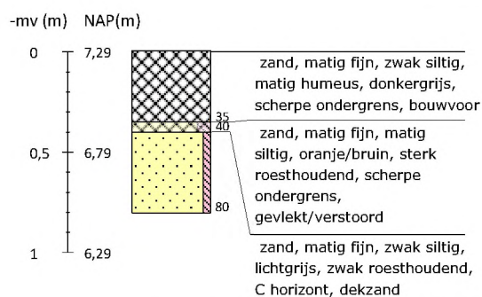
Boring 100 RD-coördinaten: 266038/550711
