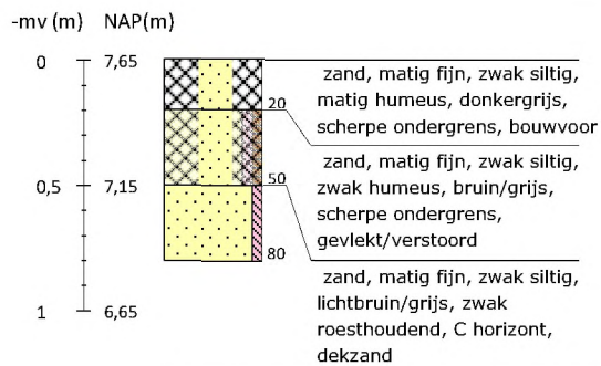
Boring 90 RD-coördinaten: 266200/550561
