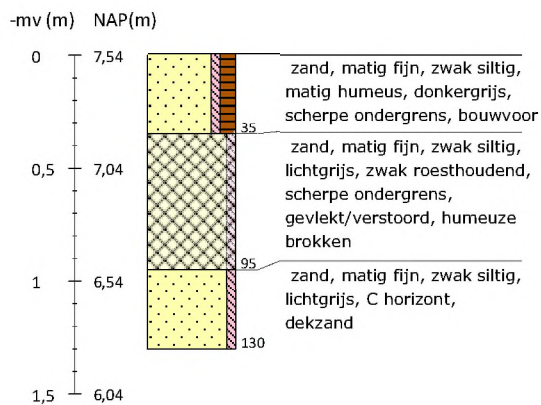
Boring 109 RD-coördinaten: 265852/551084
