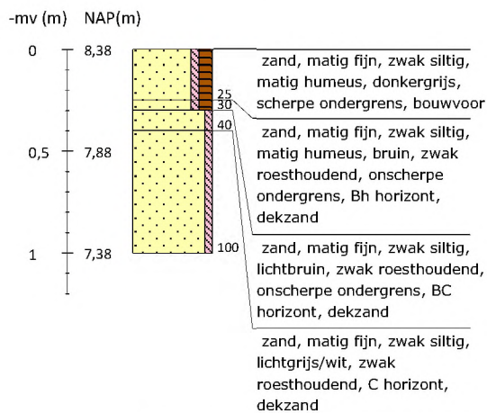
Boring 5 RD-coördinaten: 265884/550079
