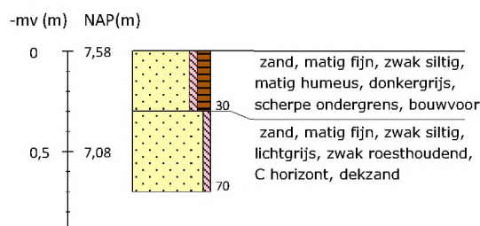
Boring 82 RD-coördinaten: 266026/550444
