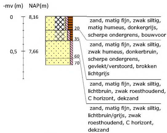
Boring 4 RD-coördinaten: 265906/550013
