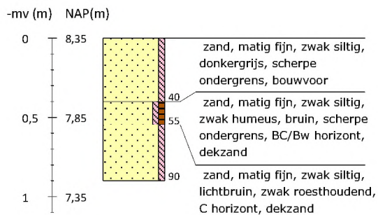
Boring 21 RD-coördinaten: 266009/549969
