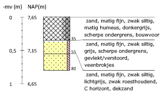
Boring 95 RD-coördinaten: 265963/550704
