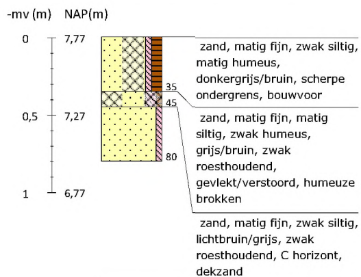
Boring 38 RD-coördinaten: 266195/550340
