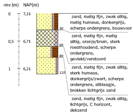
Boring 110 RD-coördinaten: 265771/551199
