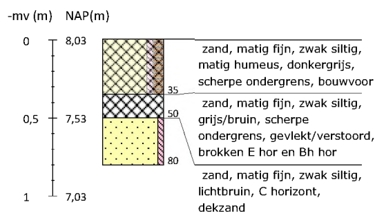
Boring 44 RD-coördinaten: 266205/550128
