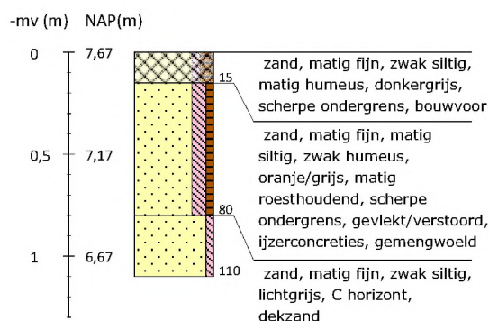
Boring 26 RD-coördinaten: 266006/550203
