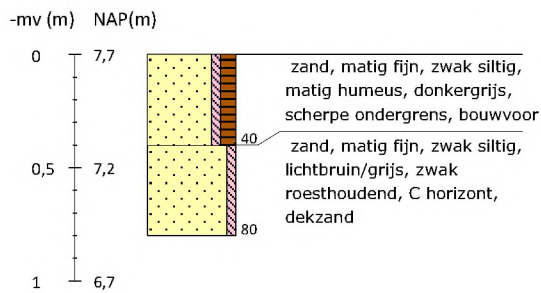
Boring 87 RD-coördinaten: 266125/550648
