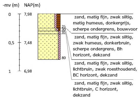
Boring 60 RD-coördinaten: 266247/550350
