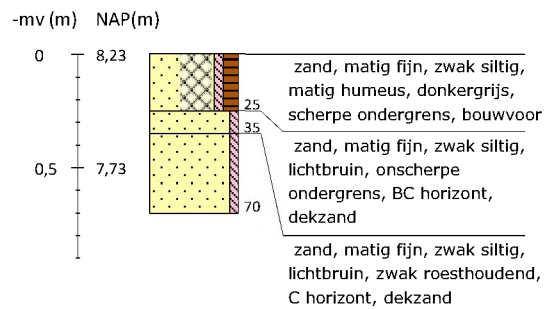
Boring 50 RD-coördinaten: 266246/550252
