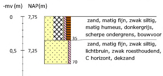
Boring 78 RD-coördinaten: 266043/550327
