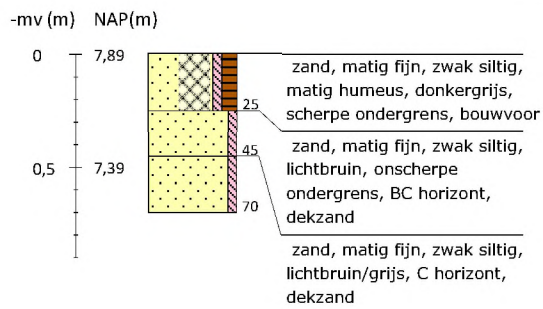
Boring 62 RD-coördinaten: 266287/550426
