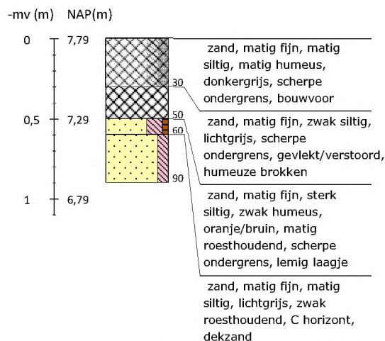
Boring 30 RD-coördinaten: 266071/549977
