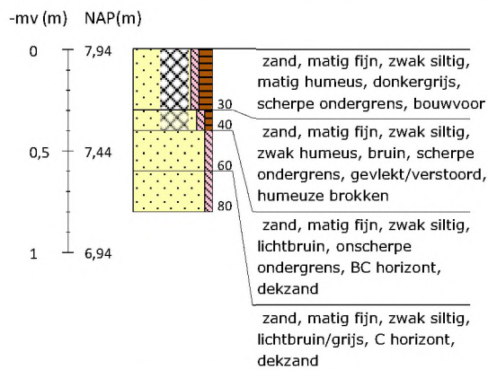
Boring 66 RD-coördinaten: 266377/550428
