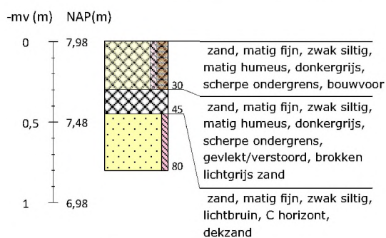
Boring 71 RD-coördinaten: 265960/550229
