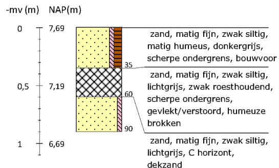
Boring 110 RD-coördinaten: 265771/551199
