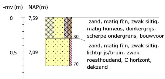
Boring 96 RD-coördinaten: 265902/550756
