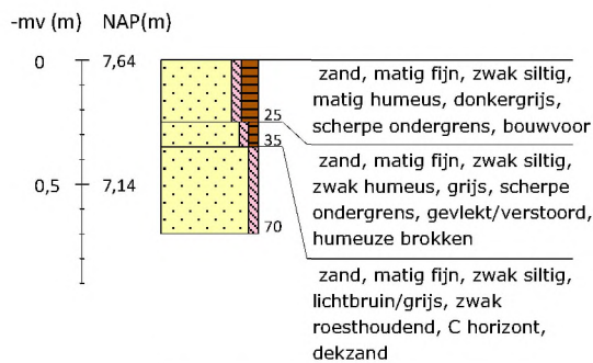
Boring 91 RD-coördinaten: 266186/550605
