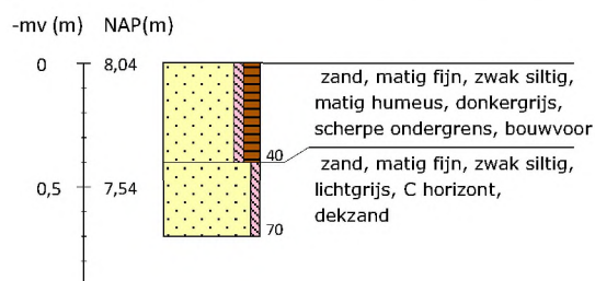
Boring 56 RD-coördinaten: 266366/550172
