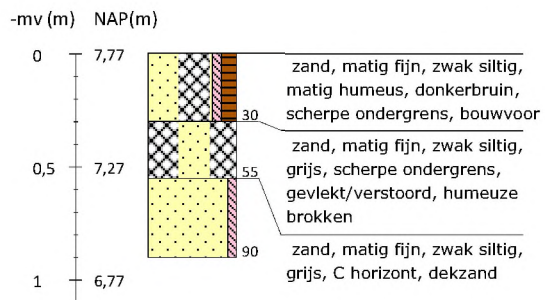
Boring 36 RD-coördinaten: 266135/550408
