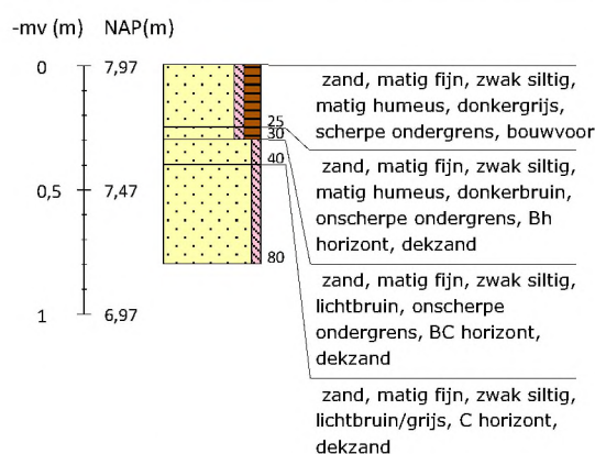
Boring 12 RD-coördinaten: 265926/550202
