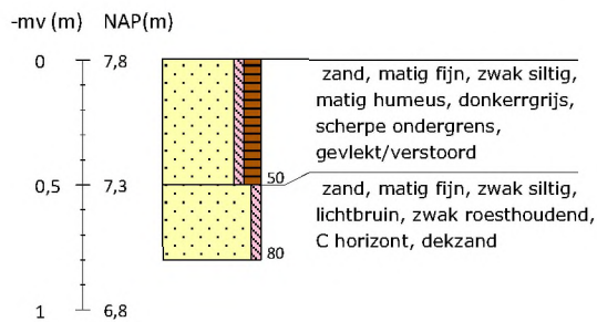
Boring 103 RD-coördinaten: 266046/550765
