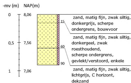
Boring 58 RD-coördinaten: 266405/550201
