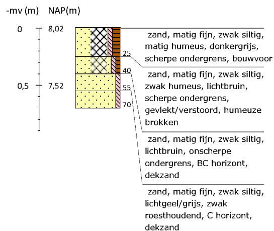
Boring 52 RD-coördinaten: 266284/550188
