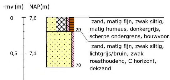
Boring 94 RD-coördinaten: 265977/550637
