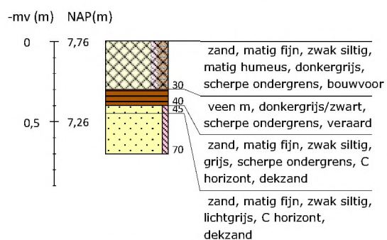
Boring 72 RD-coördinaten: 265924/550301
