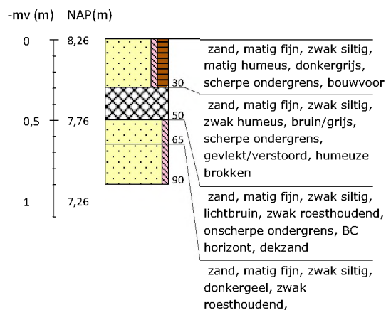
Boring 51 RD-coördinaten: 266286/550225
