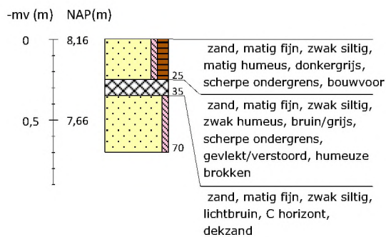
Boring 65 RD-coördinaten: 266328/550437
