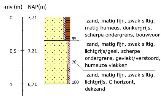
Boring 100 RD-coördinaten: 266038/550711
