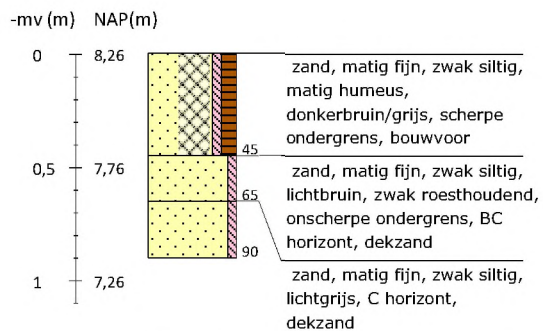
Boring 22 RD-coördinaten: 266007/550003
