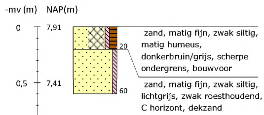
Boring 16 RD-coördinaten: 265964/550127
