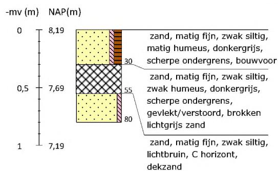
Boring 56 RD-coördinaten: 266366/550172
