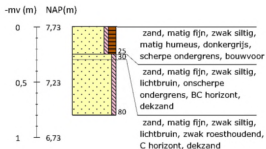
Boring 37 RD-coördinaten: 266205/550420
