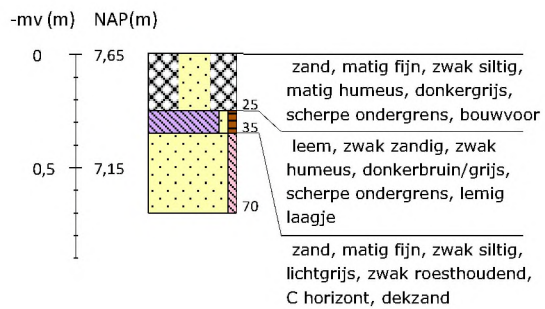
Boring 76 RD-coördinaten: 265966/550326
