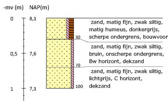
Boring 12 RD-coördinaten: 265926/550202
