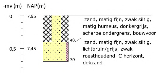
Boring 66 RD-coördinaten: 266377/550428
