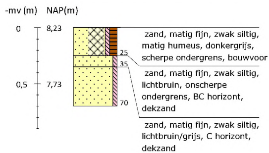
Boring 22 RD-coördinaten: 266007/550003
