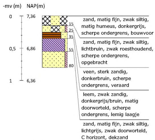
Boring 78 RD-coördinaten: 266043/550327
