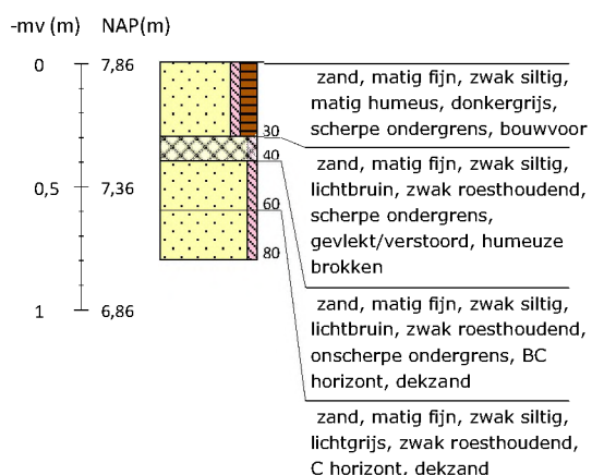
Boring 45 RD-coördinaten: 266249/550104
