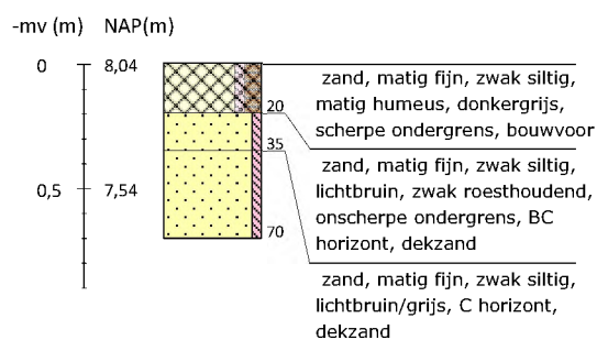
Boring 46 RD-coördinaten: 266246/550052
