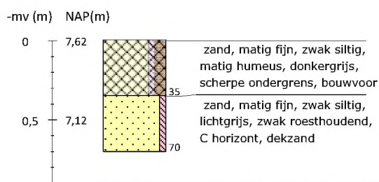
Boring 95 RD-coördinaten: 265963/550704
