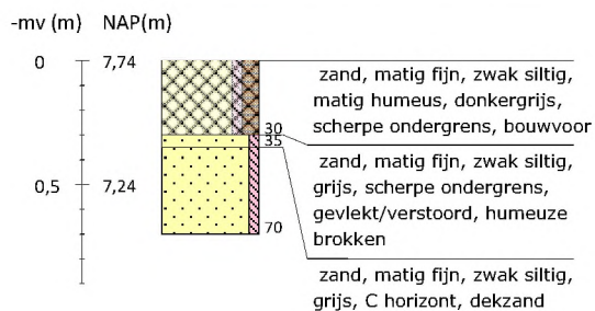
Boring 35 RD-coördinaten: 266127/550347
