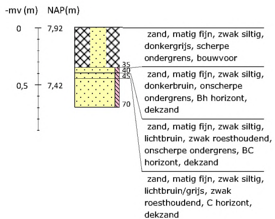
Boring 38 RD-coördinaten: 266195/550340
