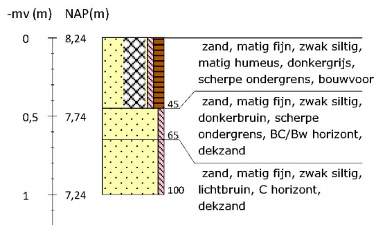
Boring 20 RD-coördinaten: 265966/549953
