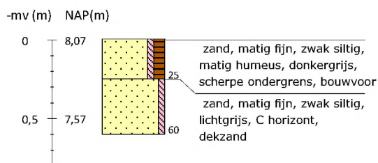
Boring 13 RD-coördinaten: 265925/550154
