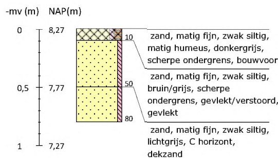
Boring 14 RD-coördinaten: 265925/550102
