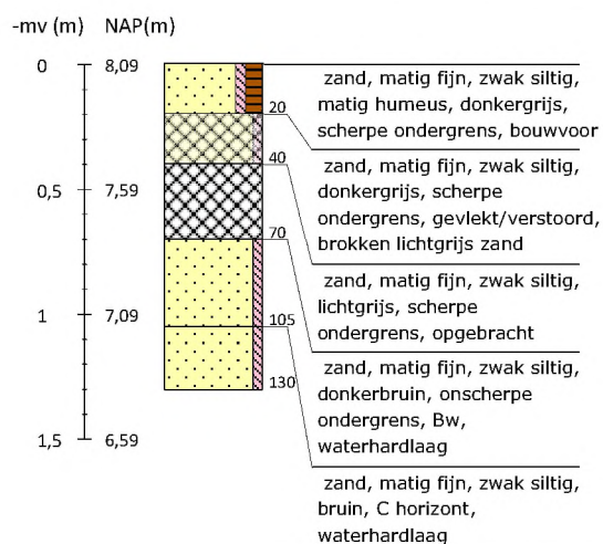
Boring 70 RD-coördinaten: 265926/550250
