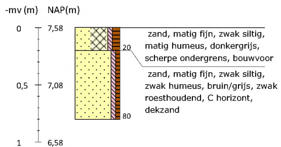
Boring 90 RD-coördinaten: 266200/550561
