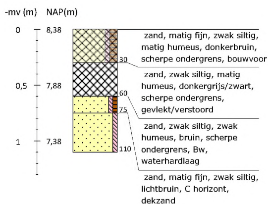
Boring 5 RD-coördinaten: 265884/550079
