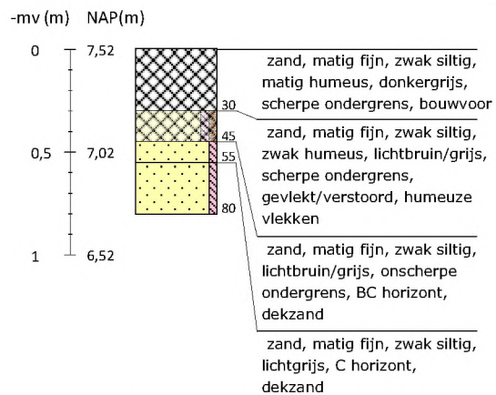
Boring 106 RD-coördinaten: 265771/550920
