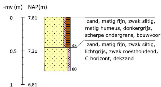
Boring 30 RD-coördinaten: 266071/549977
