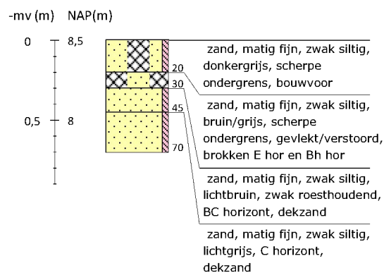
Boring 52 RD-coördinaten: 266284/550188
