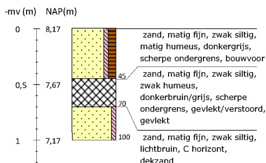
Boring 25 RD-coördinaten: 266007/550148
