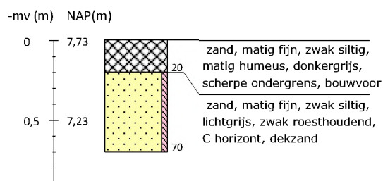
Boring 44 RD-coördinaten: 266205/550128
