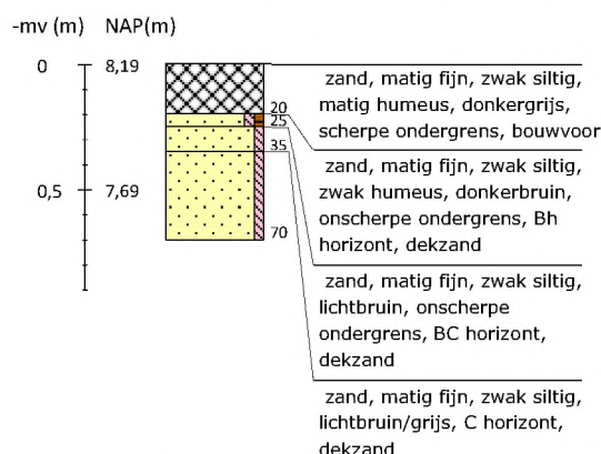
Boring 10 RD-coördinaten: 265886/550227
