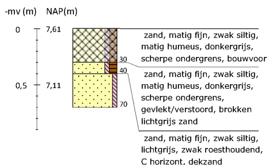
Boring 43 RD-coördinaten: 266206/550079
