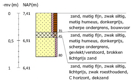
Boring 108 RD-coördinaten: 265868/551042
