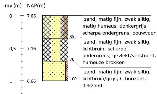
Boring 34 RD-coördinaten: 266132/550271
