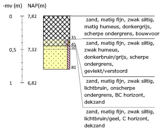
Boring 63 RD-coördinaten: 266286/550376
