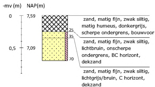
Boring 107 RD-coördinaten: 265793/551002
