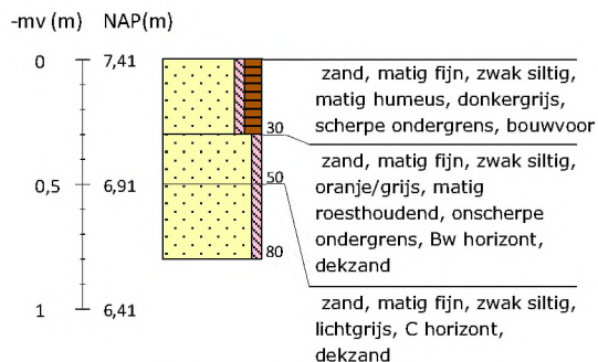
Boring 109 RD-coördinaten: 265852/551084
