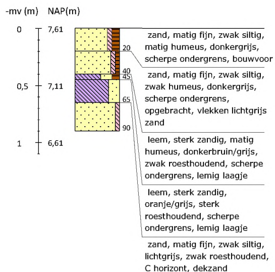
Boring 72 RD-coördinaten: 265924/550301
