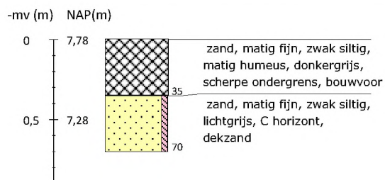
Boring 102 RD-coördinaten: 266084/550790
