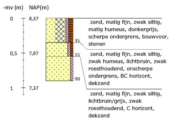
Boring 6 RD-coördinaten: 265886/550128
