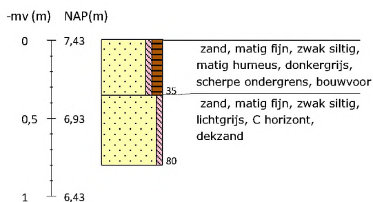
Boring 97 RD-coördinaten: 265837/550782
