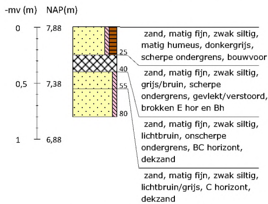
Boring 65 RD-coördinaten: 266328/550437
