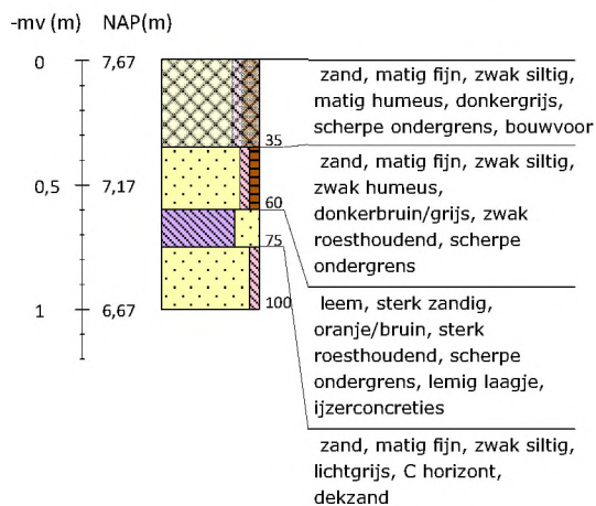
Boring 29 RD-coördinaten: 266048/550070
