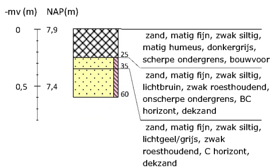
Boring 41 RD-coördinaten: 266169/550104
