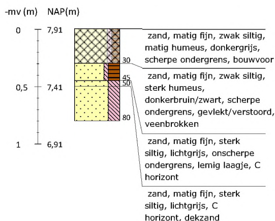
Boring 27 RD-coördinaten: 266049/550253
