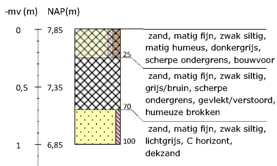
Boring 45 RD-coördinaten: 266249/550104
