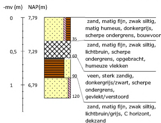
Boring 86 RD-coördinaten: 266077/550632
