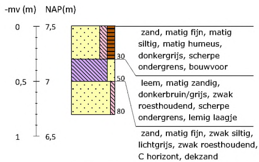
Boring 75 RD-coördinaten: 265945/550390
