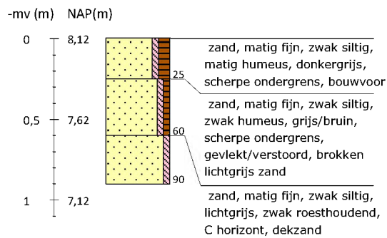
Boring 49 RD-coördinaten: 266246/550200
