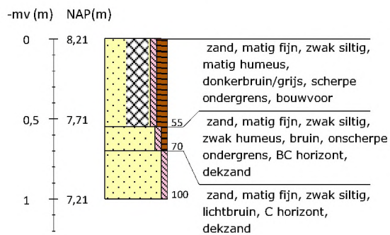
Boring 4 RD-coördinaten: 265906/550013
