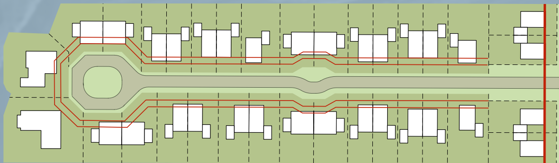
Figuur 22. De woningen worden op 4 tot 7 meter van de kavelgrens geplaatst in de woonstraat, aan de Horsa staan de woningen op een vaste rooilijn
