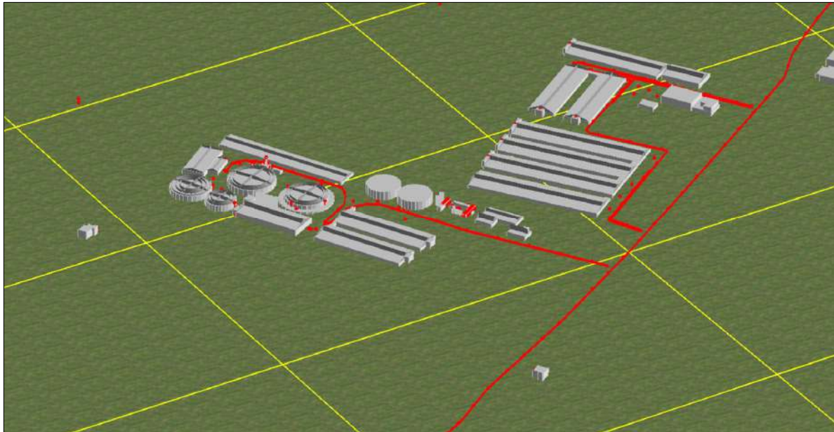
Afbeelding 2: 3D-weergave van het rekenmodel (RBS, gezien vanuit zuidwestelijke richting)
