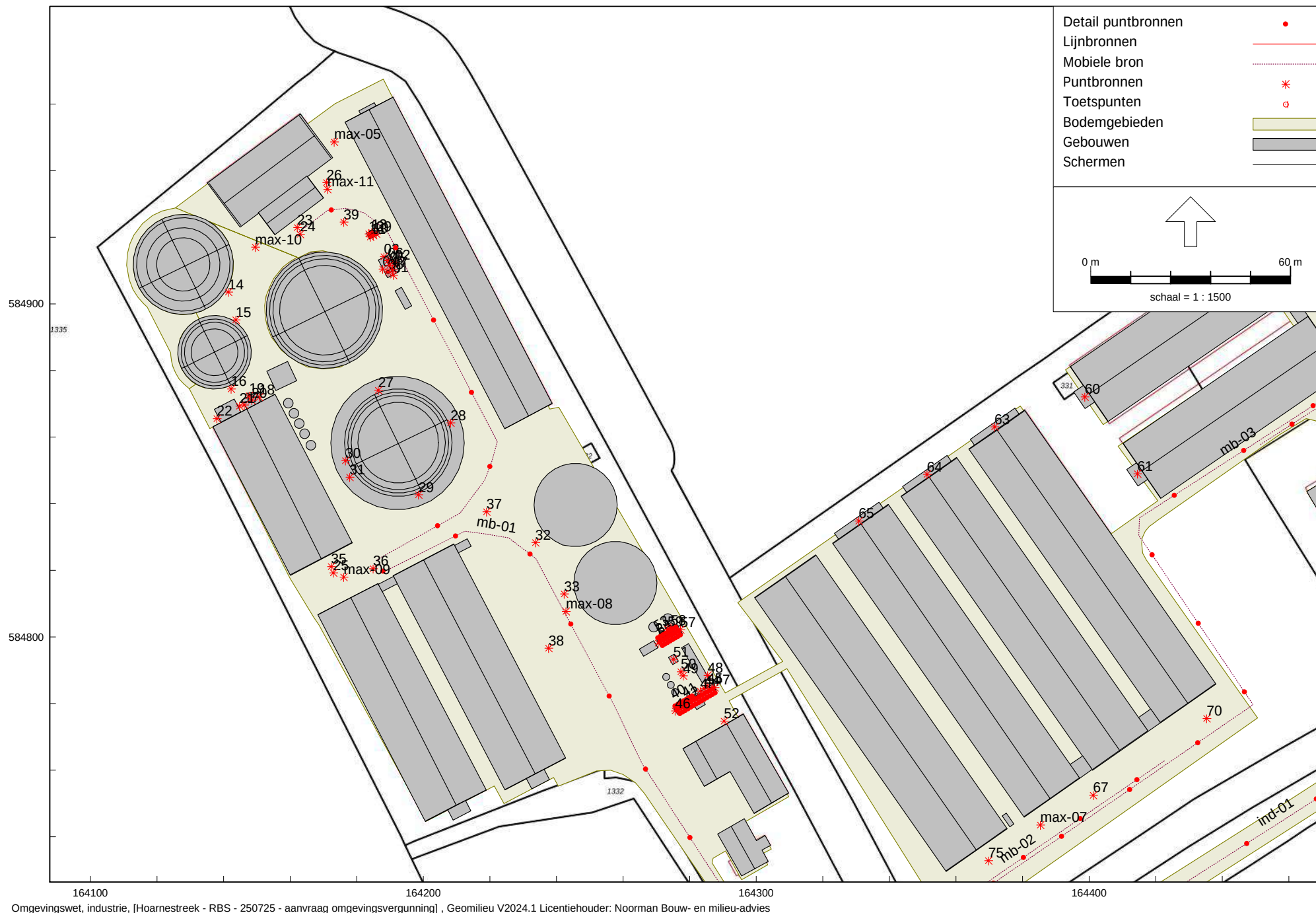
RBS: Detailoverzicht van het rekenmodel incl. geluidbronnen
