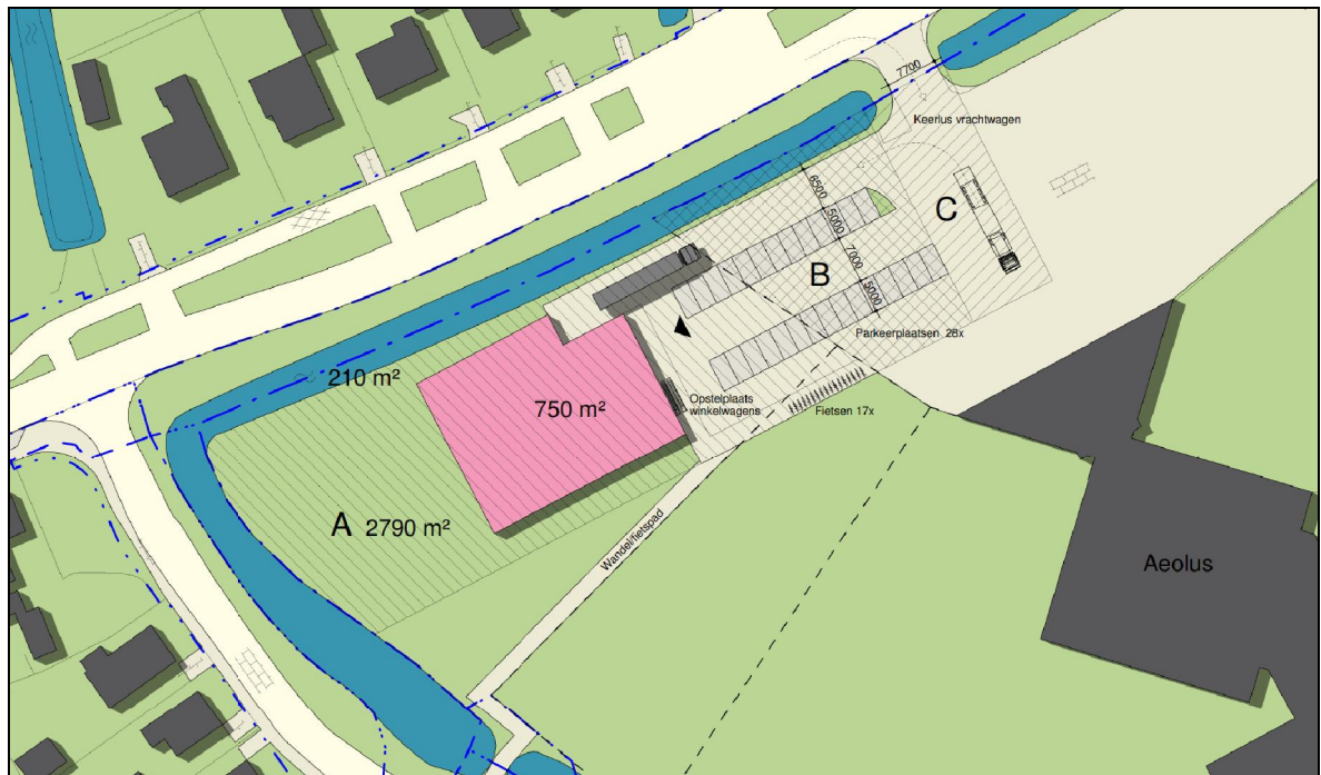
Figuur 3. Plansituatie Hearewei 24 te Sexbierum.
