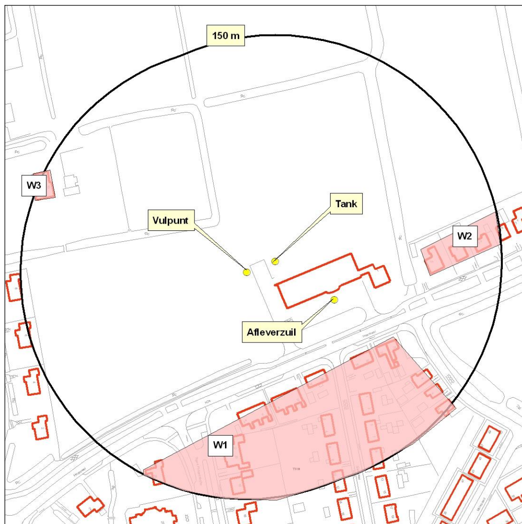
Figuur 2. Omgeving LPG-tankstation huidige situatie
