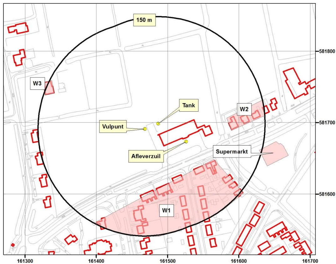
Figuur 3. Omgeving LPG-tankstation toekomstige situatie
