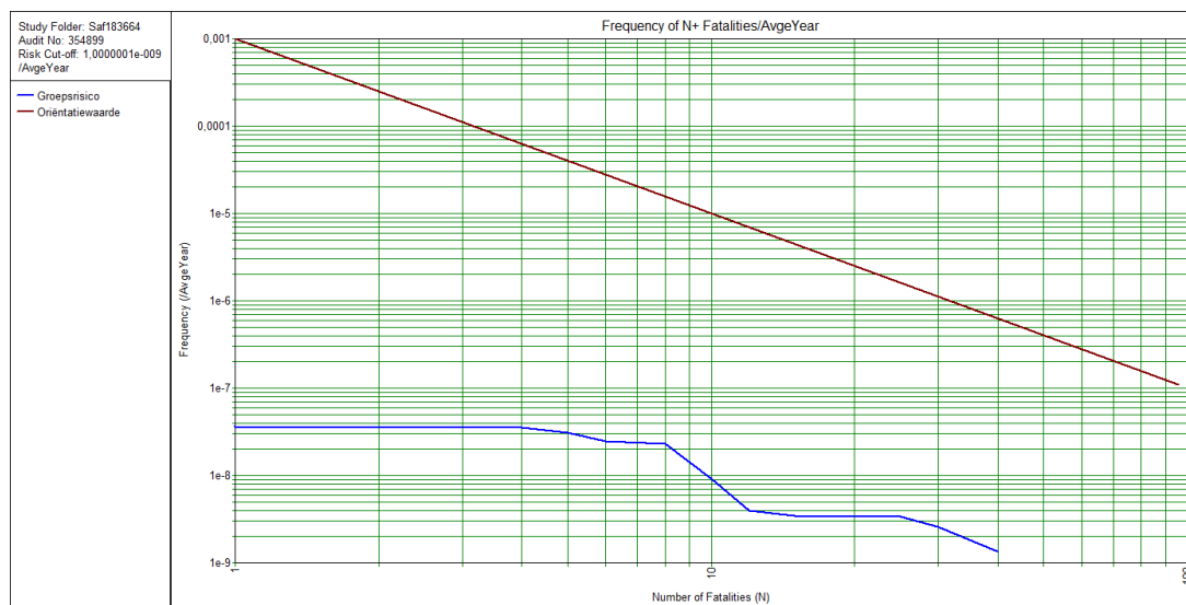
Figuur 5. Groepsrisico huidige situatie bij doorzet tot 1000 m 3 /jr
