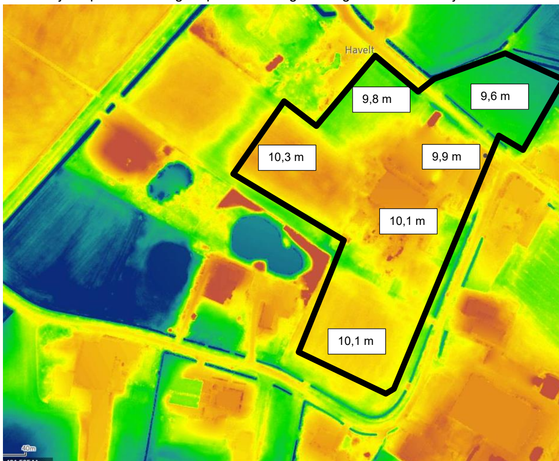
Figuur 7. Hoogteverschil onderzoekslocatie (bron: Ahn)
