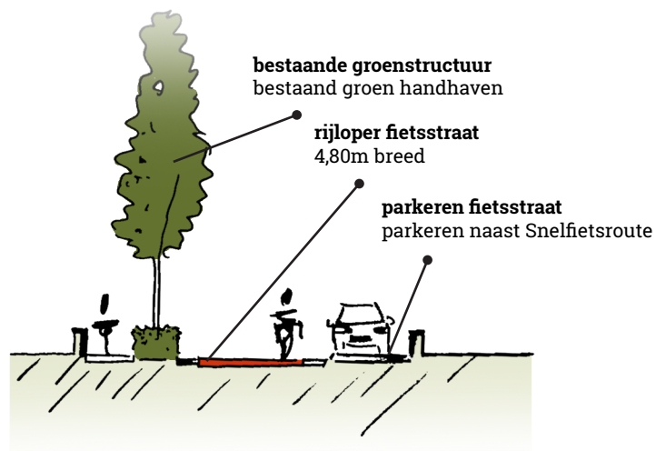
Principeschets fietsstraat (Burg. Schrevensingel, Geerbosch, Spoorven, Rietven, Moerven en Turfven Veghel)
