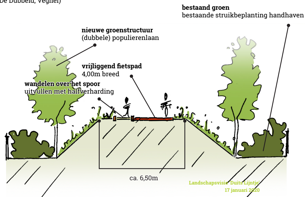
Principeschets vrijliggend fietspad 'talud Gazellebrug' bedrijventerrein (De Dubbeld, Veghel)
