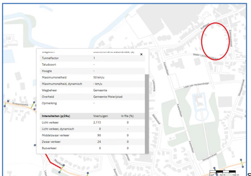
Afbeelding 6. Verkeersgegevens CIMLK met de verkeersintensiteit van het met rood gemarkeerde wegvak (Zuidelijke Randweg). De ligging van het plangebied is met rood omcirkeld.
