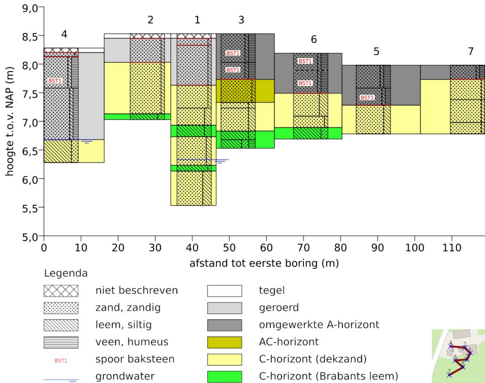
Figuur 28: Boorprofielen.
