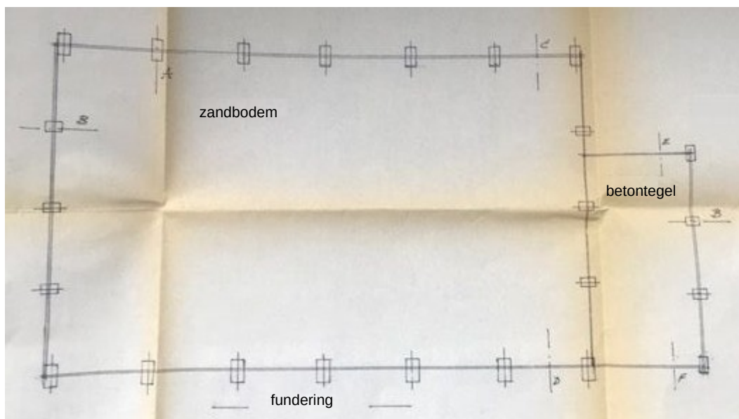
Figuur 8: Funderingsplan uit 1990 van de zuidelijke (te slopen) loods.
