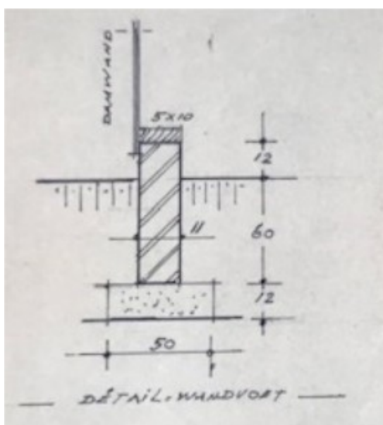
Figuur 9: Detail fundering zuidelijke loods.
