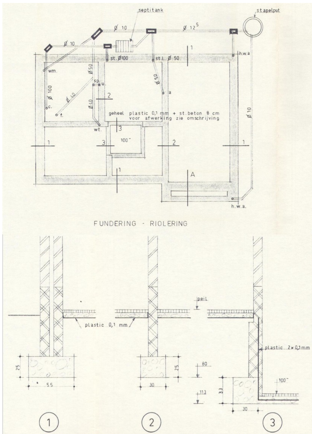
Figuur 10: Bouwtekening woonhuis en doorsnede funderingen (noorden linksonder).
