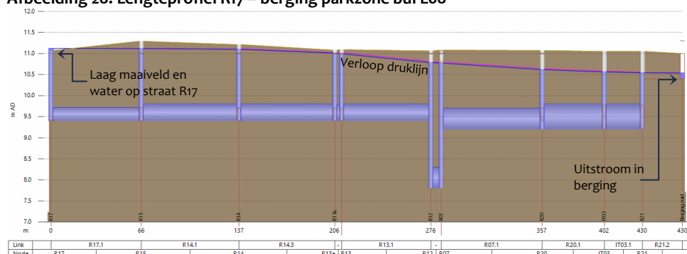
Afbeelding 28: Lengteprofiel R17 – berging parkzone bui L08
