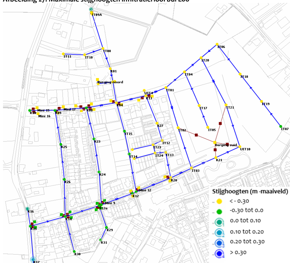
Afbeelding 27: Maximale stijghoogten infiltratierool bui L08
