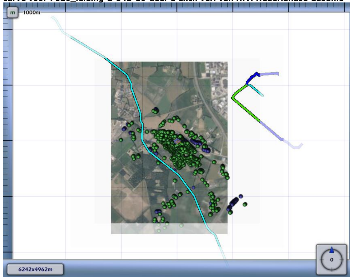
Figuur 4.2 Kilometer leiding behorende bij de maximale overschrijding van de FN-curve voor 7126_leiding-Z-542-10-deel-1 excl. verl van N.V. Nederlandse Gasunie
