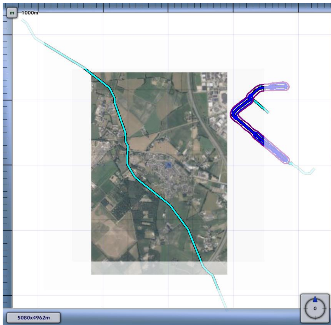
3.4 Figuur 3.4 Plaatsgebonden risico voor 7130_leiding-Z-542-10-deel-1 incl. verl van N.V. Nederlandse Gasunie
