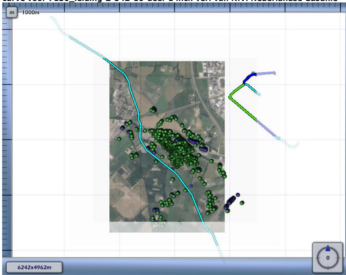
Figuur 4.4 Kilometer leiding behorende bij de maximale overschrijding van de FN-curve voor 7130_leiding-Z-542-10-deel-1 incl. verl van N.V. Nederlandse Gasunie
