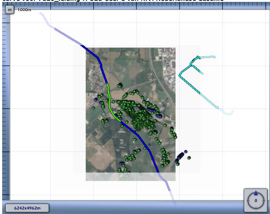
Figuur 4.1 Kilometer leiding behorende bij de maximale overschrijding van de FN-curve voor 7126_leiding-A-521-deel-1 van N.V. Nederlandse Gasunie
