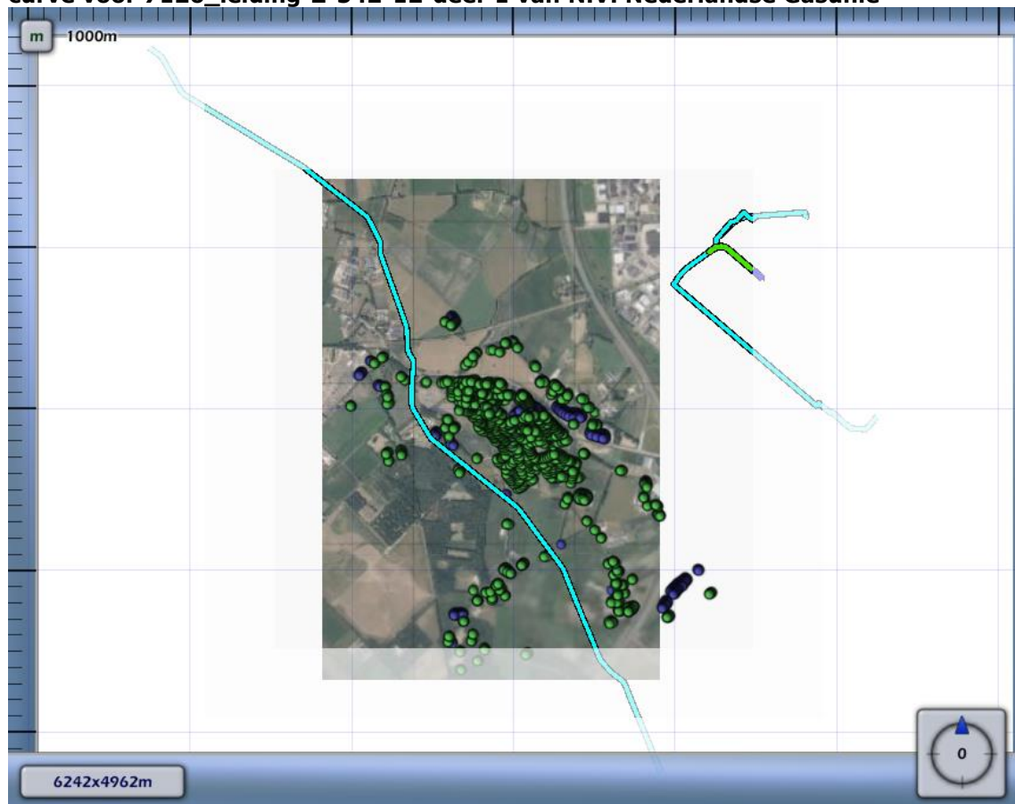
Figuur 4.3 Kilometer leiding behorende bij de maximale overschrijding van de FN-curve voor 7126_leiding-Z-542-12-deel-1 van N.V. Nederlandse Gasunie
