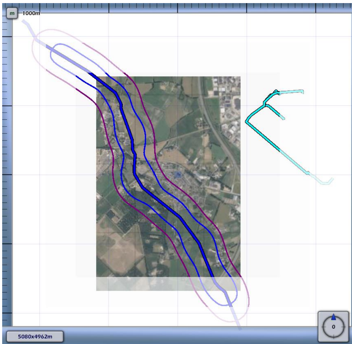
3.1 Figuur 3.1 Plaatsgebonden risico voor 7126_leiding-A-521-deel-1 van N.V. Nederlandse Gasunie
