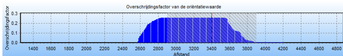
Afbeelding 3 Groepsrisico screening A-521-deel1 huidige situatie ter hoogte van het plangebied
