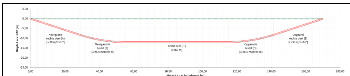
Figuur 2.11: Boorprofiel verbinding tussen winputten en zuiveringsinstallatie.
