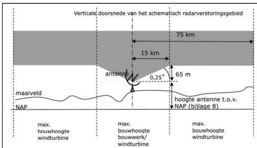
Figuur 3.1: Schematische weergave radarverstoringsgebied.
