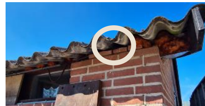
Figuur 10: Opening tussen bolling van golfplaten en gevel van opstal
