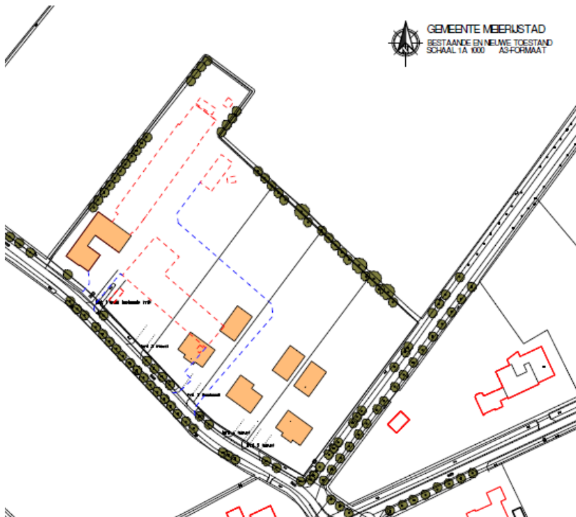
Figuur 4. Onderzoekslocatie met schets bouwplan
