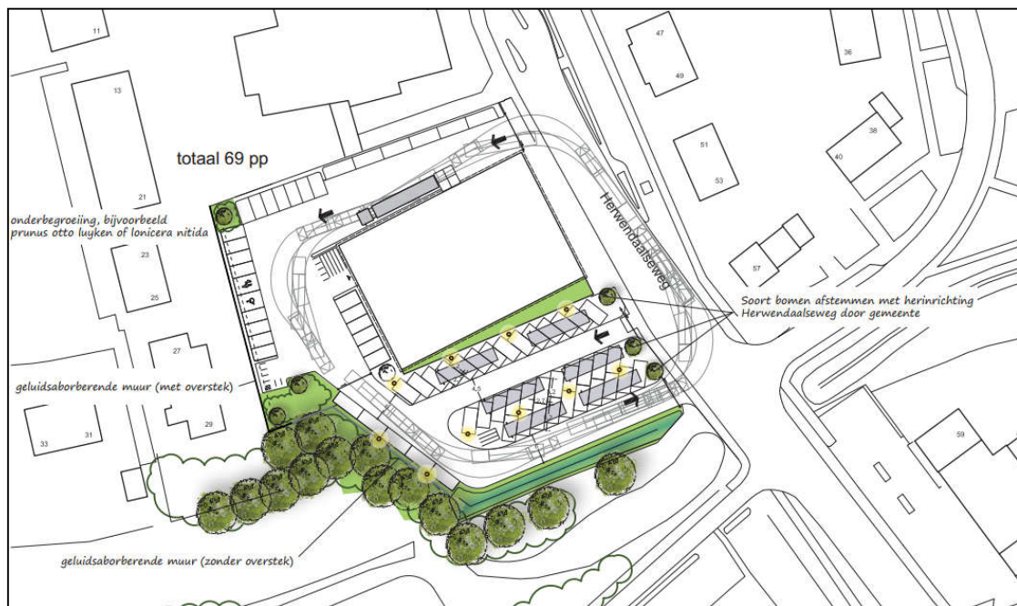
Figuur 1: Overzicht schetsontwerp inrichting parkeerterrein Lidl Groesbeek (bron: BRO).
