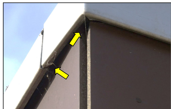
Figuur 8. Voorbeeld van opening tussen daktrim en boeiboord
