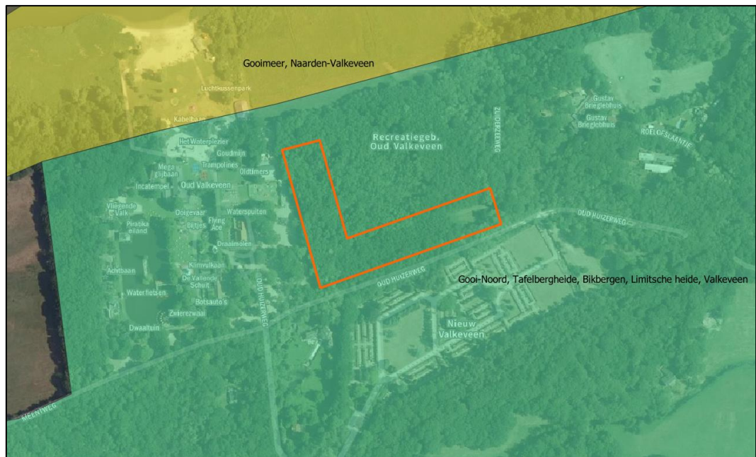
Figuur 3.6 Aardkundige waarden in en nabij de locatie van het zoekgebied (oranje arcering). De aardkundige waarden zijn ingedeeld in deelgebieden (groene en gele vlak). Bron: Provincie Noord-Holland (2019); bron achtergrond: PDOK.
