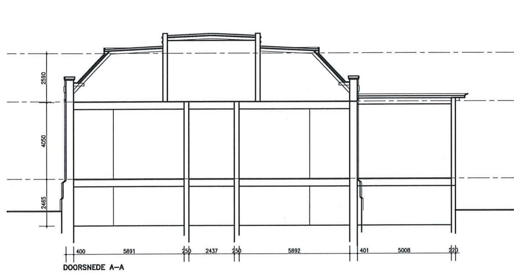
DOORSNEDE A-A
