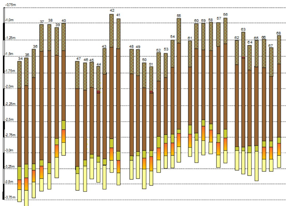
Figuur 10: Lemmer, Lemsterhoek: De boringen 34 tot en met 68 in de vorm van boorprofielen.
