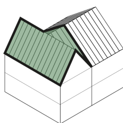
Nokverdraaiing toepassen op prominente plekken
