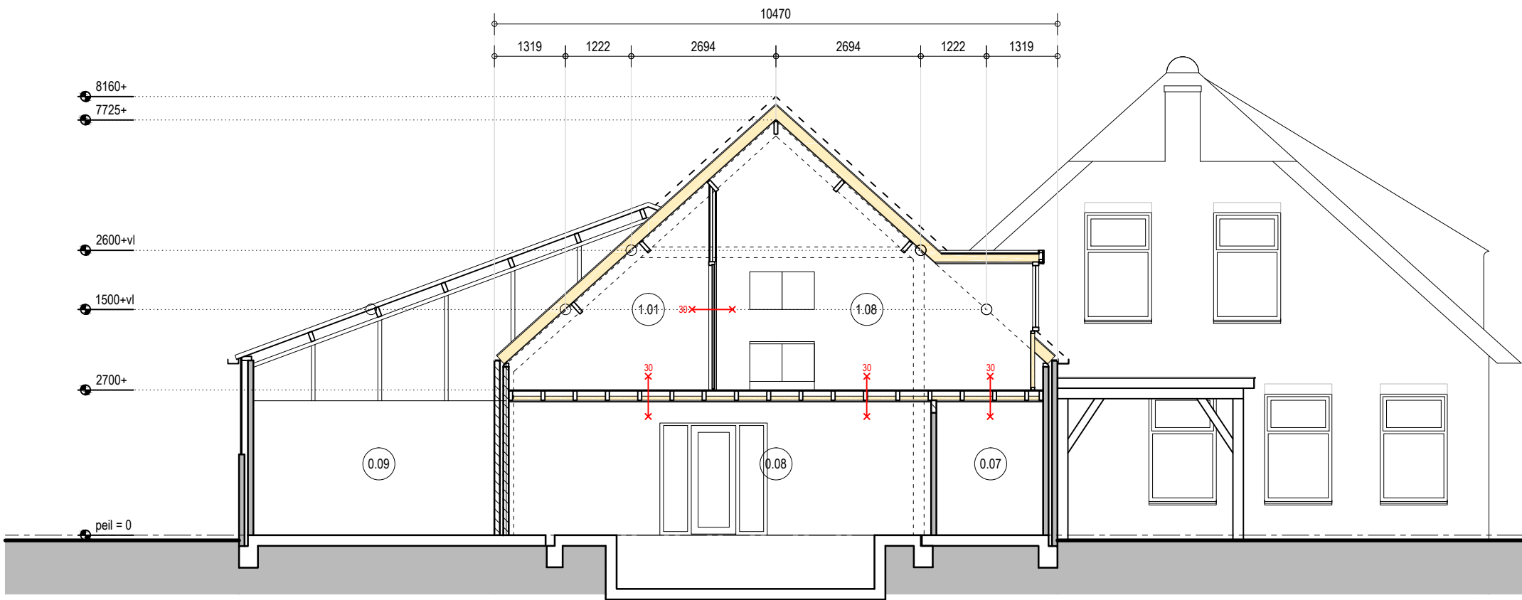
doorsnede: A
