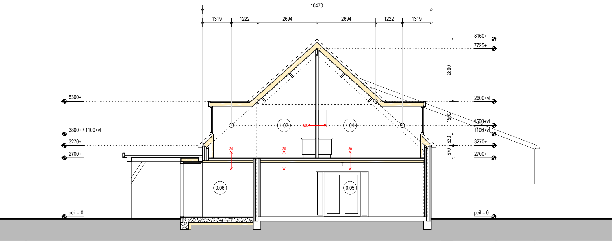
doorsnede: B
