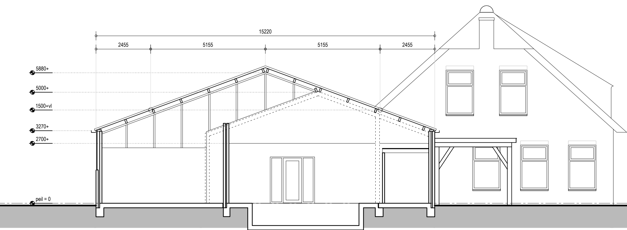
doorsnede: A
