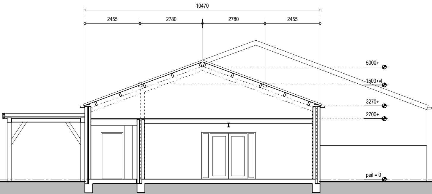
doorsnede: B
