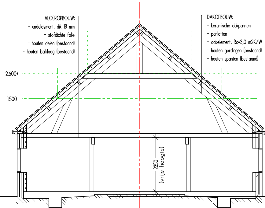
DOORSNEDE C bestaand
