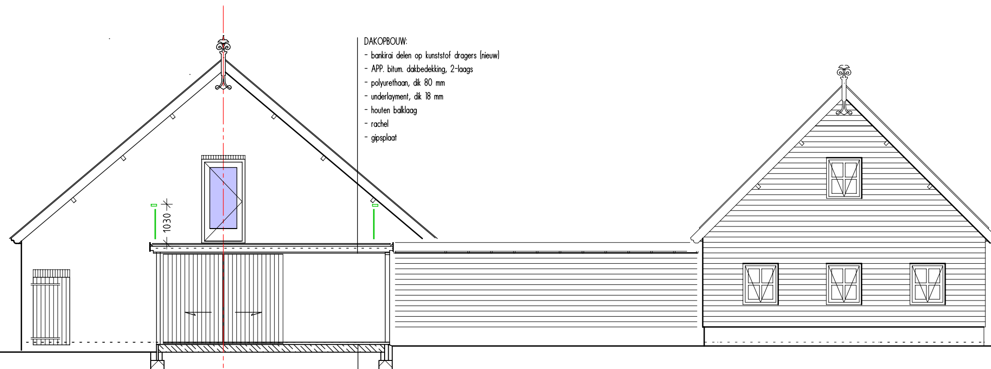
DOORSNEDE C gewijzigd
