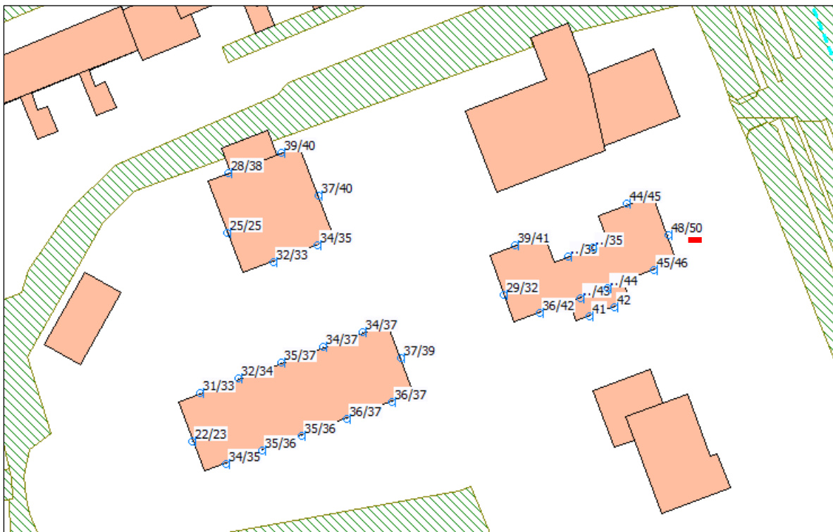
Figuur 3: Geluidsbelasting vanwege de Bredeweg (incl. aftrek ex art. 110g van 5 dB) op de woningen binnen het plangebied.
