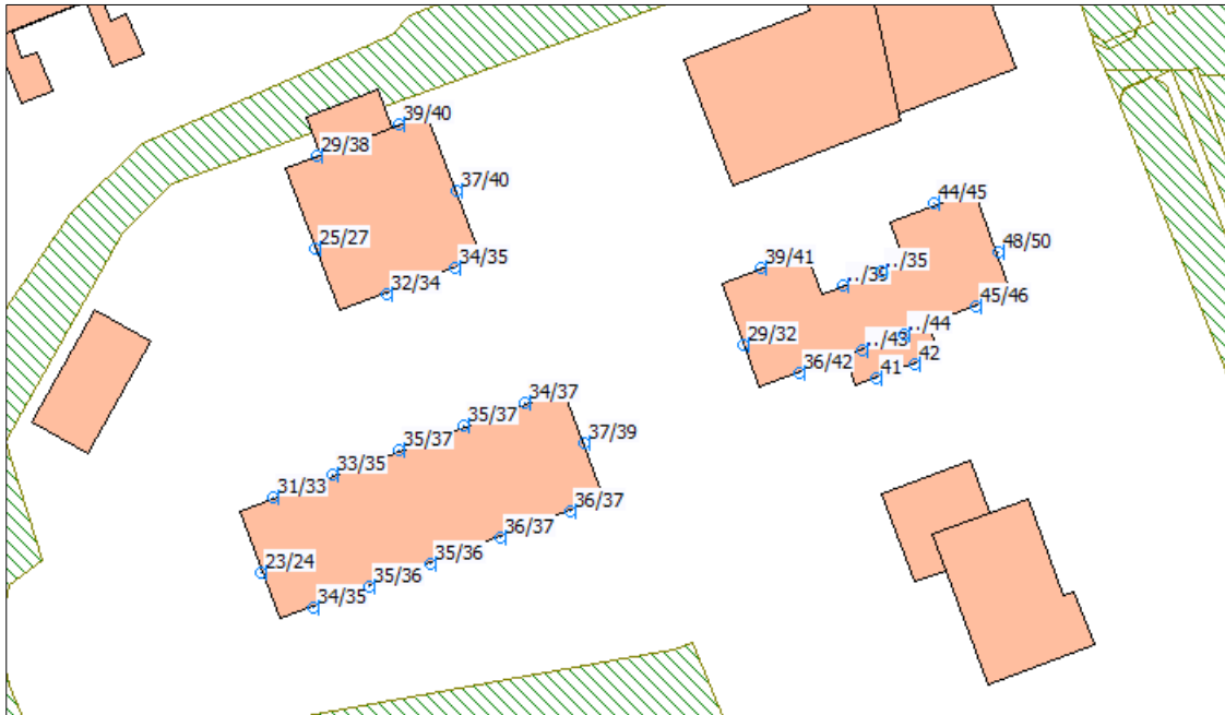
Figuur 4: Gecumuleerde geluidsbelasting excl. aftrek ex art. 110g
