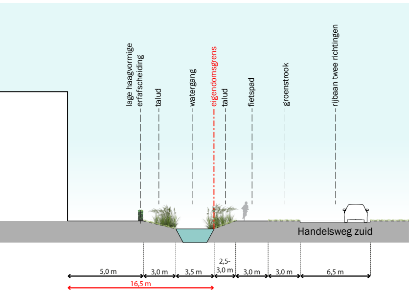
Profiel D - Handelsweg zuid
