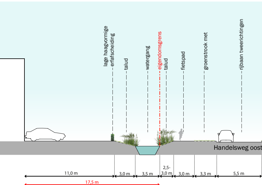
Profiel C - Handelsweg oost
