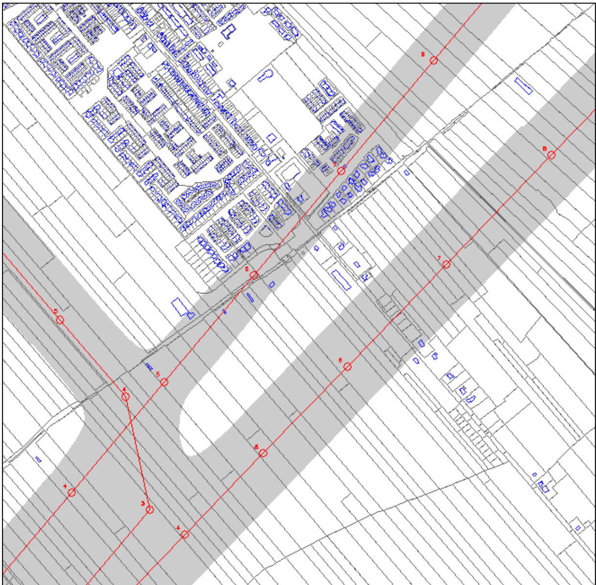
Figuur 8: Specifieke magneetveldzone ter hoogte van Ouderkerk a/d IJssel
