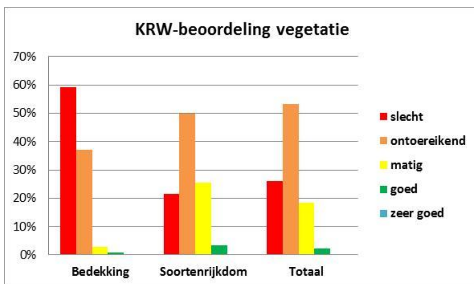
Figuur 4.14 KRW-beoordeling van water- en oeevervegetatie op basis van de landelijke meetlat van gebufferde veensloten of van een veenkanaal (bron: HHSK).
