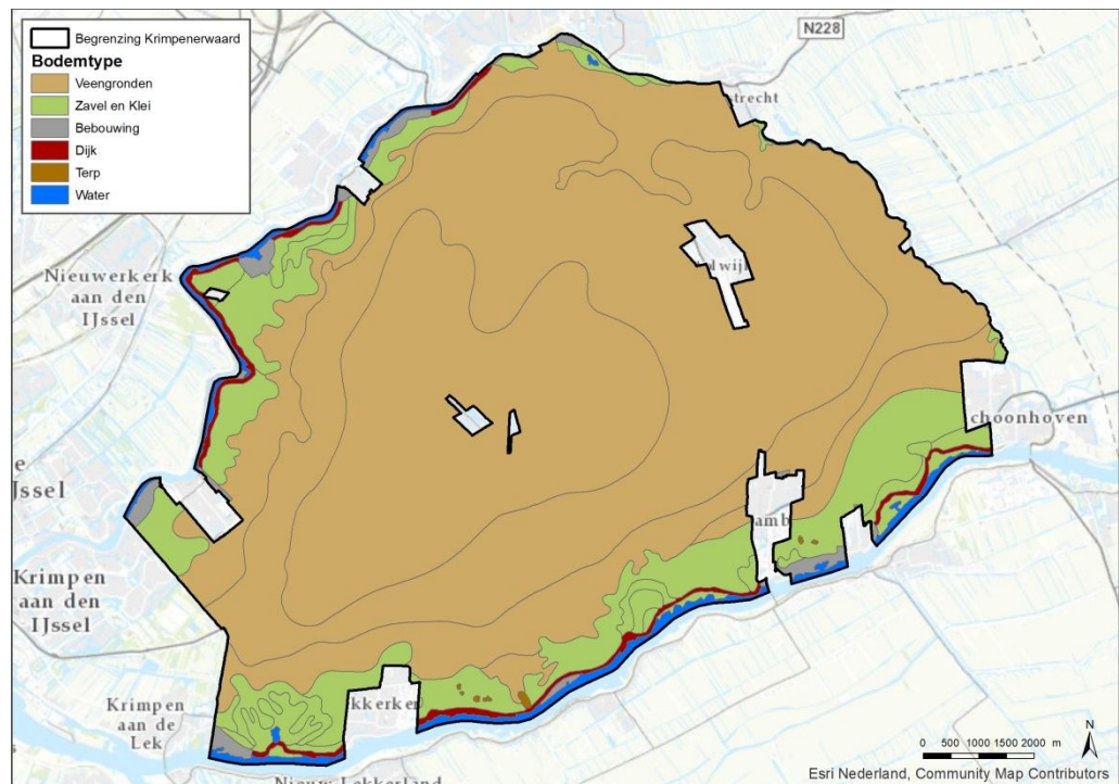
Figuur 3.6 Bodemkaart Krimpenerwaard.
