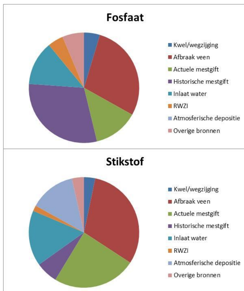
Figuur 3.5 Overzicht oorzaken voedselrijkdom oppervlaktewater (Schipper e.a., 2016).
