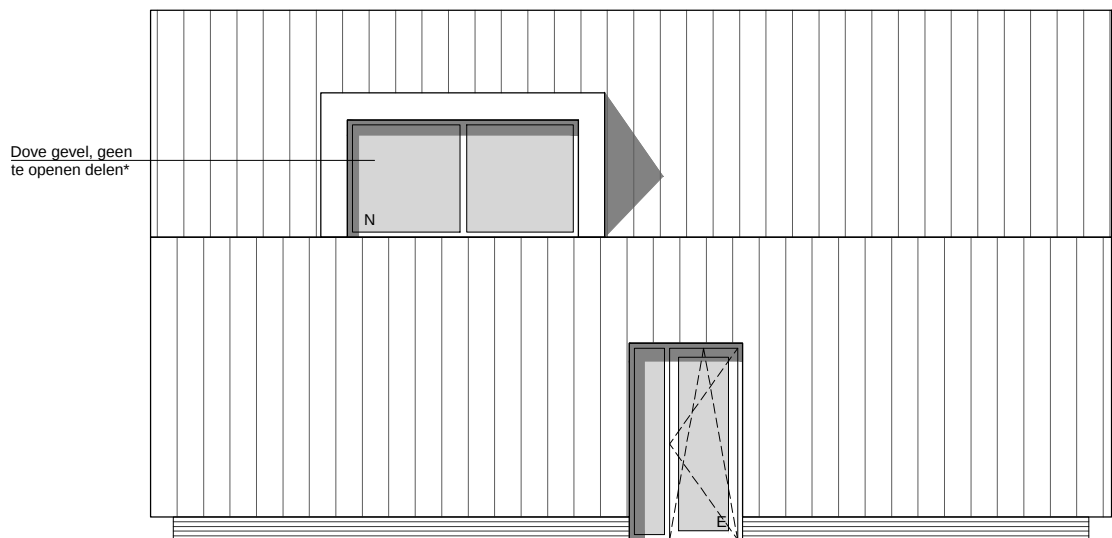
Linker zijgevel (noordzijde)
