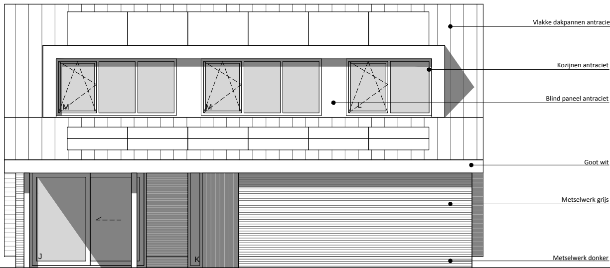
Rechter zijgevel (zuidzijde)
