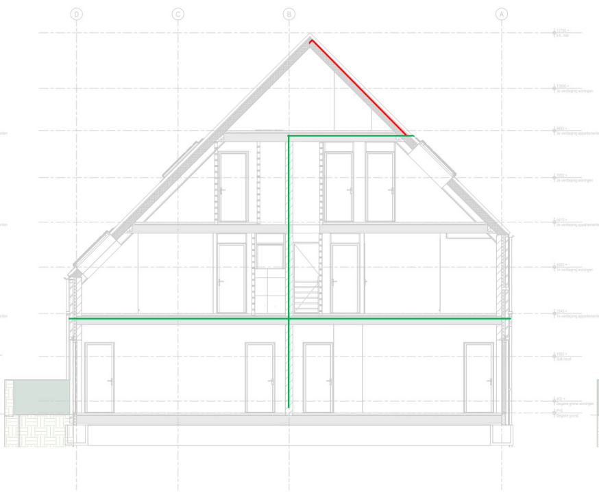
Doorsnede B
