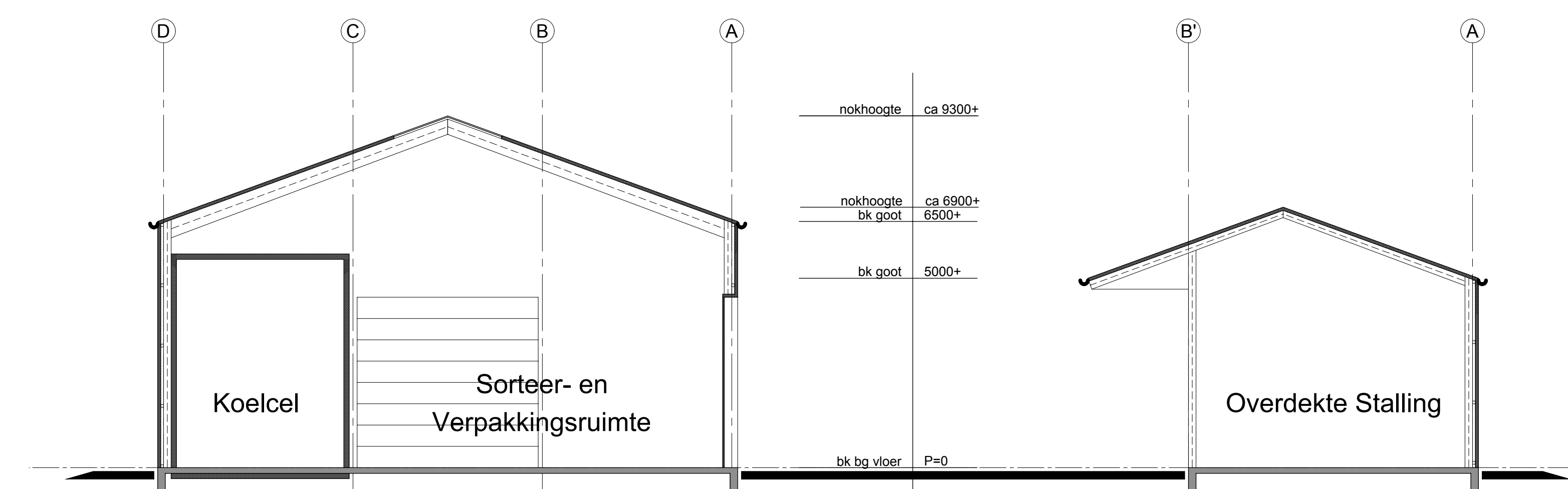
Doorsnede A
