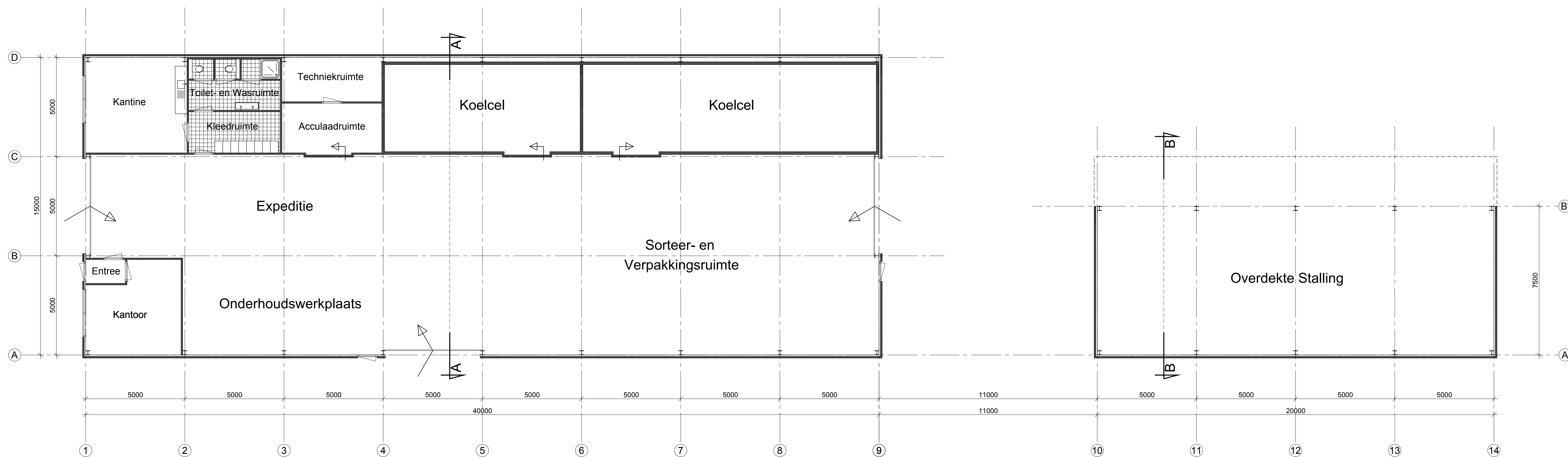
Begane Grond
