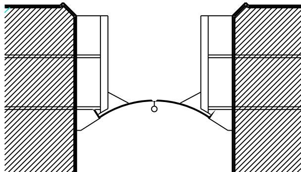
(weg) profiel 3 schaal 1:100
