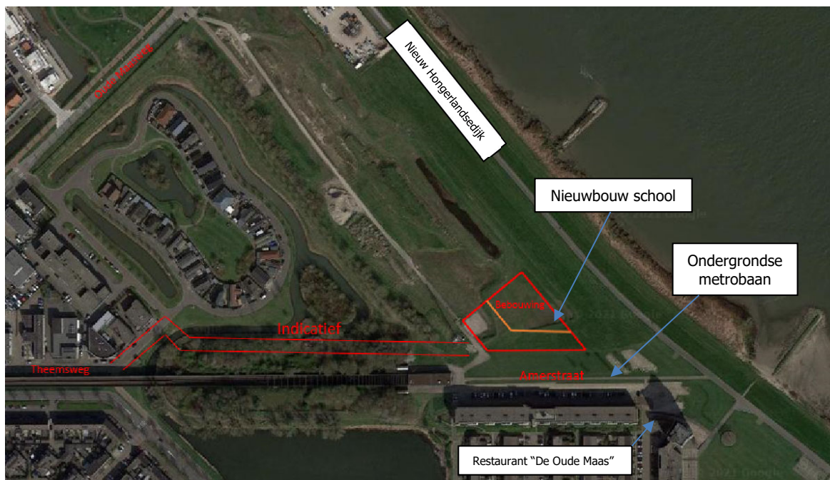
Figuur 2.1 Situatie nieuwbouwplan
