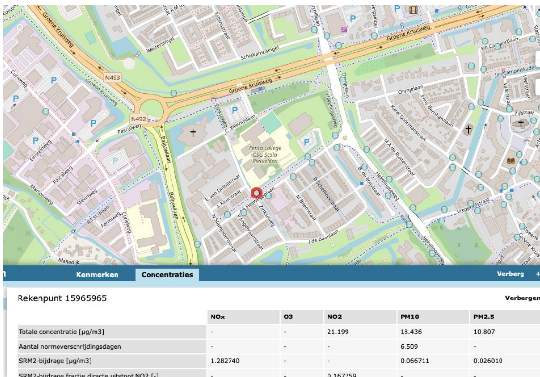
Figuur 4.6 NSL-monitoringstool
