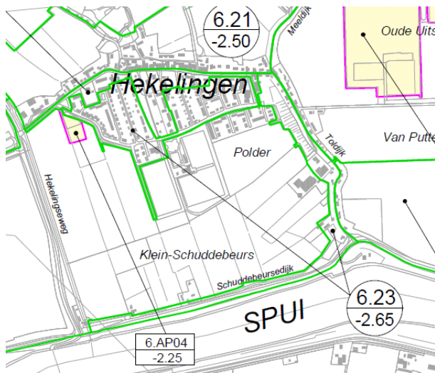
Figuur 4.5 tekening peilgebied
