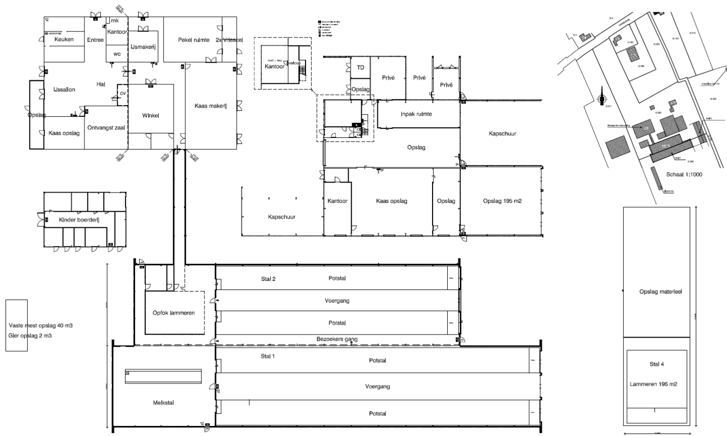
Figuur 3 Overzichtstekening bedrijf
