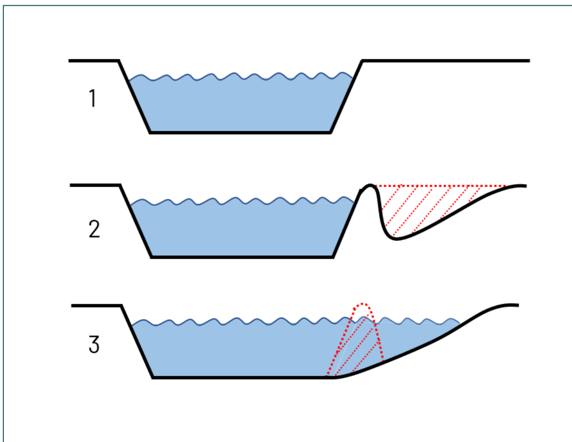
Figuur 1 Weergave van de werkwijze van de te realiseren watergangen. Eerst wordt de nieuwe watergang geheel gerealiseerd met een dam om het water tegen te houden. Als de nieuwe watergang helemaal is gerealiseerd kan de dam verwijderd worden.
