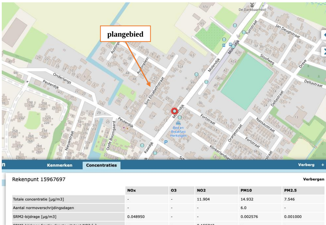
Figuur 4.1: concentraties luchtkwaliteit op rekenpunt 15967697 nabij Sint Elizabethstraat
