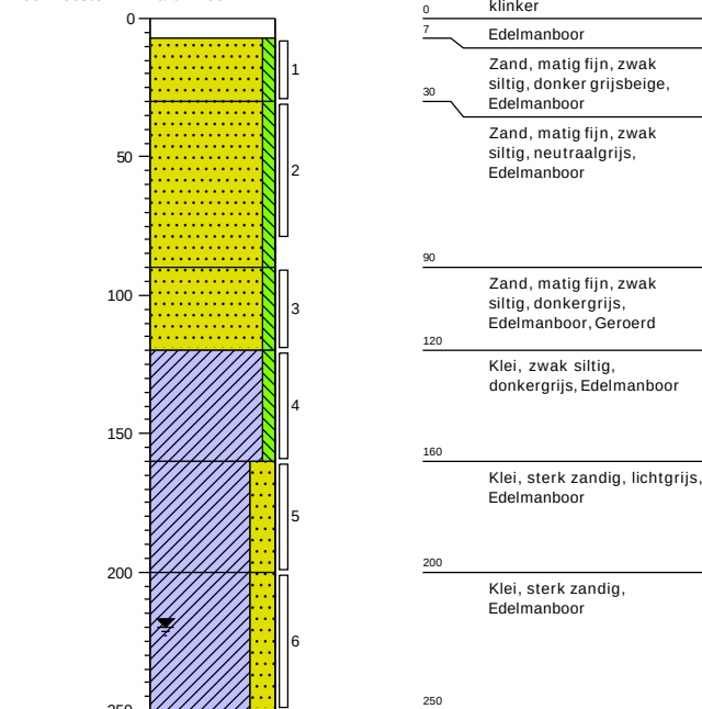
Boring: 4 Datum: 8-9-2022 Boormeester: Martin Boer
