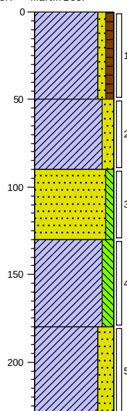
Boring: 18 Datum: 8-9-2022 Boormeester: Martin Boer
