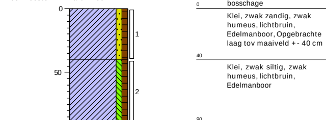
Boring: 8 Datum: 8-9-2022 Boormeester: Martin Boer
