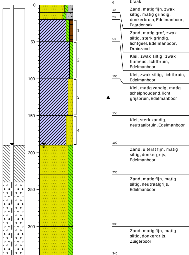
Boring: 3 Datum: 8-9-2022 Boormeester: Martin Boer
