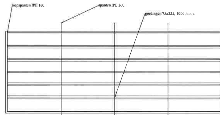
KAPPLAN
