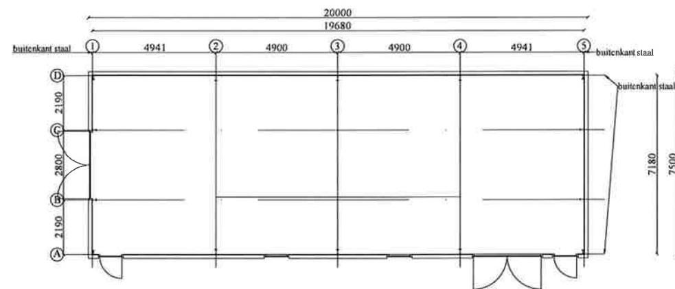
PLATTEGROND
