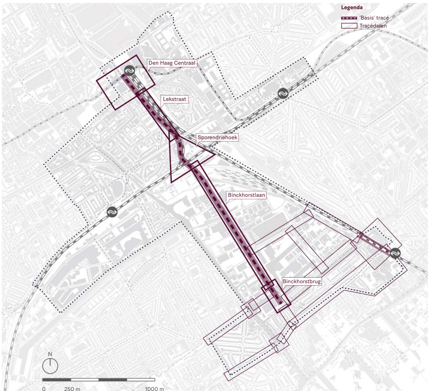
Figuur 56: Overzicht tracédelen van 'basis' tracé
