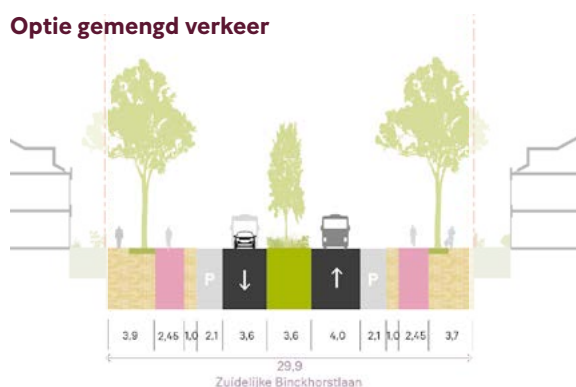
Figuur 63: Dwarsprofiel Voorburgse Binckhorstlaan
