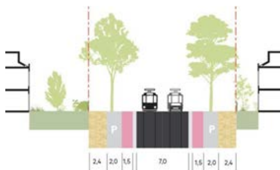
Figuur 85: Dwarsprofiel Prinses Mariannelaan voor (HOV)tram
