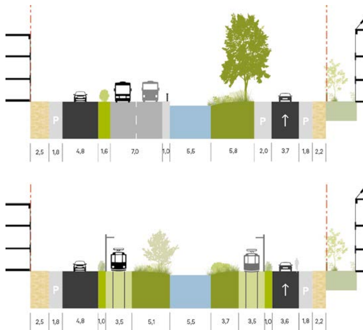
Figuur 89: Dwarsprofiel Broekslootkade voor HOV-bus en HOV-tram
