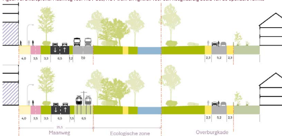
Figuur 77: Dwarsprofiel Maanweg voor HOV-bus en HOV-tram, optie HOV-baan buiten de ecologische zone
