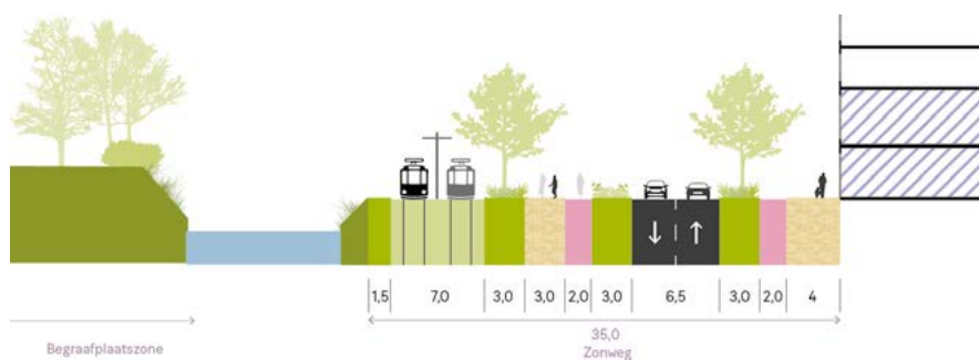
Figuur 37: Dwarsprofiel Zonweg voor HOV-tram
