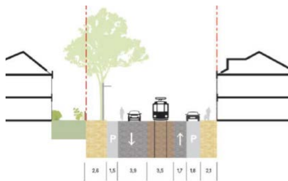
Figuur 47: Dwarsprofiel Laan van Middenburg voor tram
