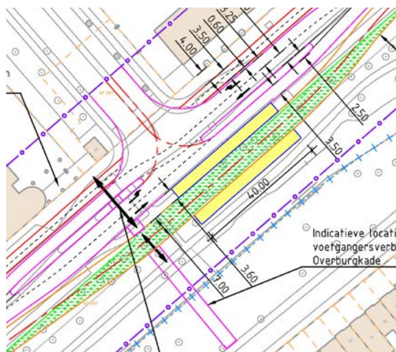
Figuur 78: Halte bij kruispunt Maanweg-Melkwegstraat
