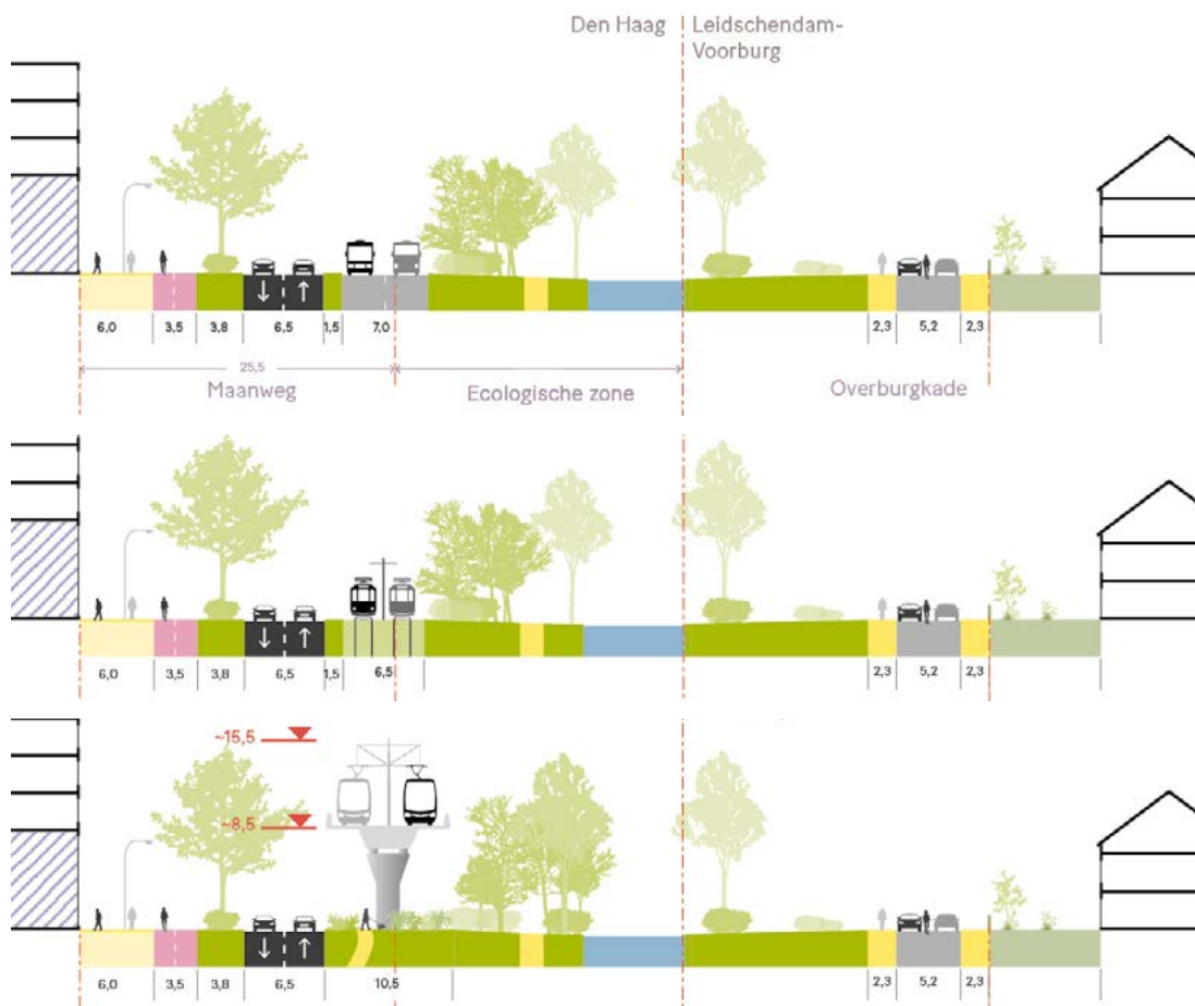
Figuur 76: Dwarsprofiel Maanweg voor HOV-bus, HOV-tram en lightrail voor een hoogwaardig beeld van de openbare ruimte
