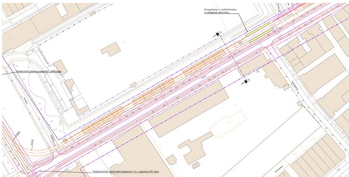
Figuur 79: Inpassing HOV-baan in de Zonweg
