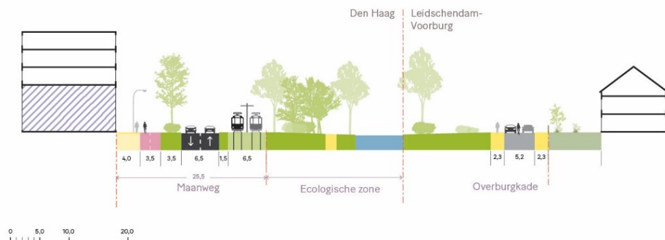
Figuur 4.8: Dwarsprofiel en impressie schetsontwerp HOV-tram Maanweg (Den Haag) met behoud van de groenzone
