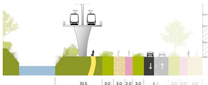
Figuur 81: Dwarsprofiel Zonweg voor HOB-bus, HOV-tram en lightrail
