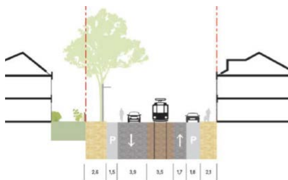
Figuur 86: Dwarsprofiel Laan van Middenburg voor tram
