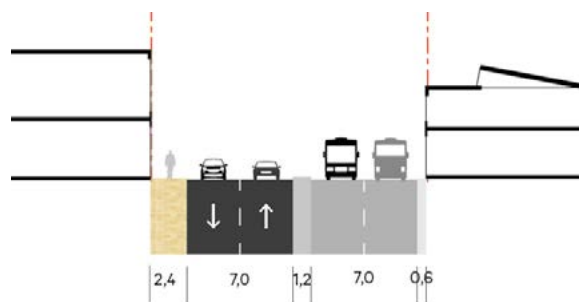
Figuur 84: Dwarsprofiel Melkwegstraat voor HOV-bus nabij de Zonweg
