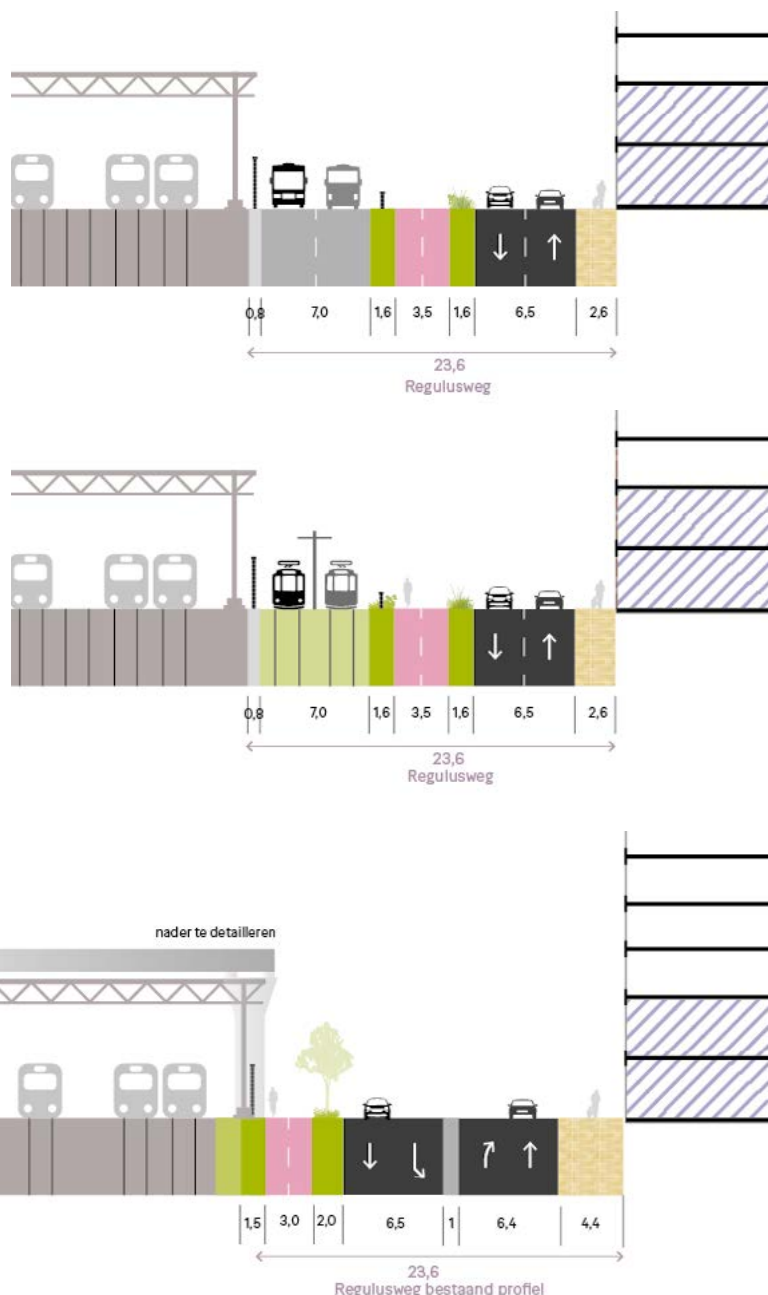
Figuur 83: Dwarsprofiel van inpassing HOV-baan in de Regulusweg bij HOV-bus, HOV-tram en lightrail (indicatief)
