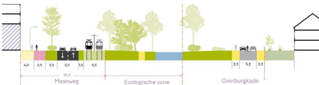
Figuur 95: Dwarsprofiel Maanweg voor HOV-bus en HOV-tram, optie HOV-baan buiten de ecologische zone
