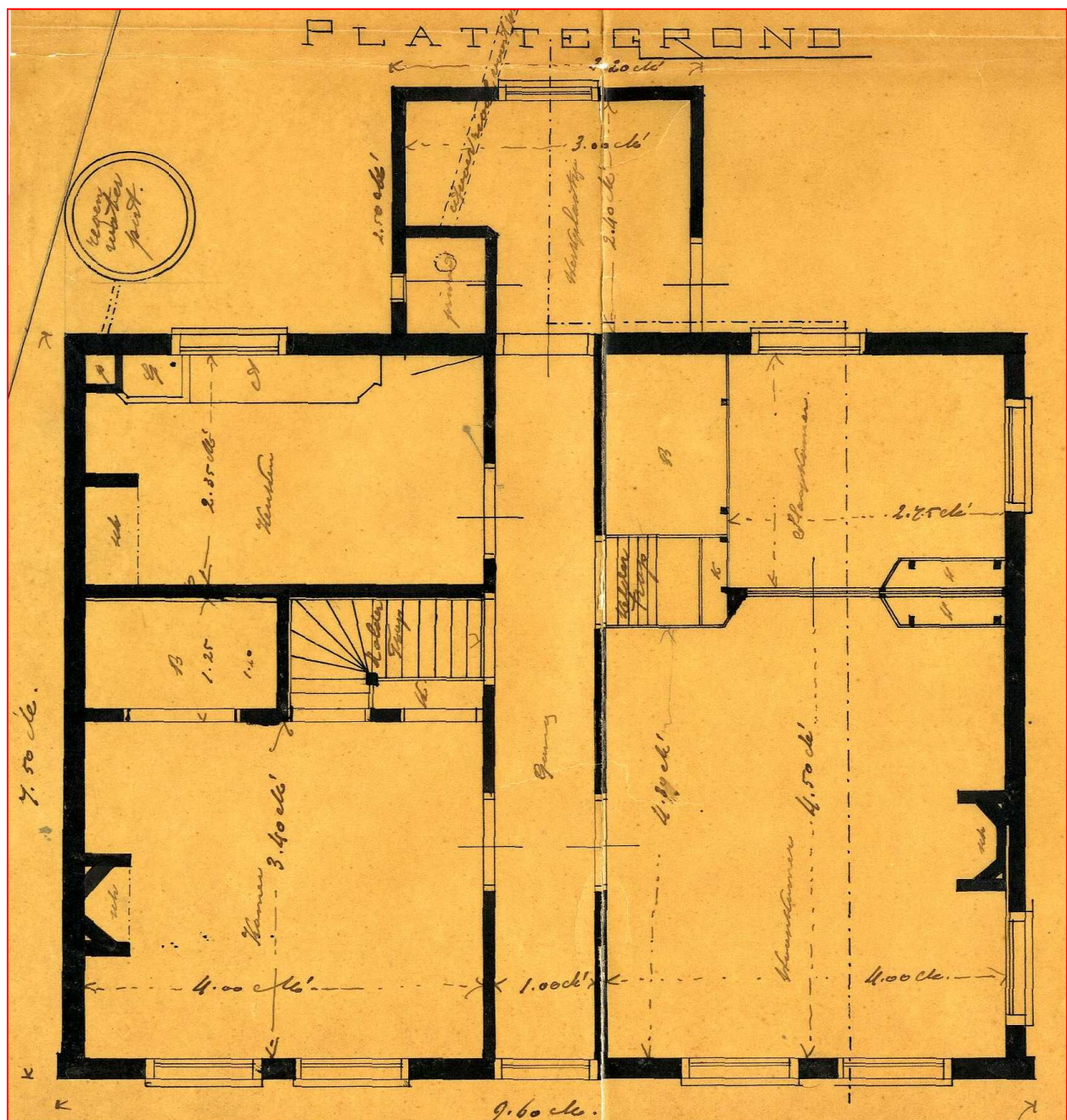
Bouwtekening behorend bij de in 1904 verleende bouwvergunning, Oostvlietweg 39
