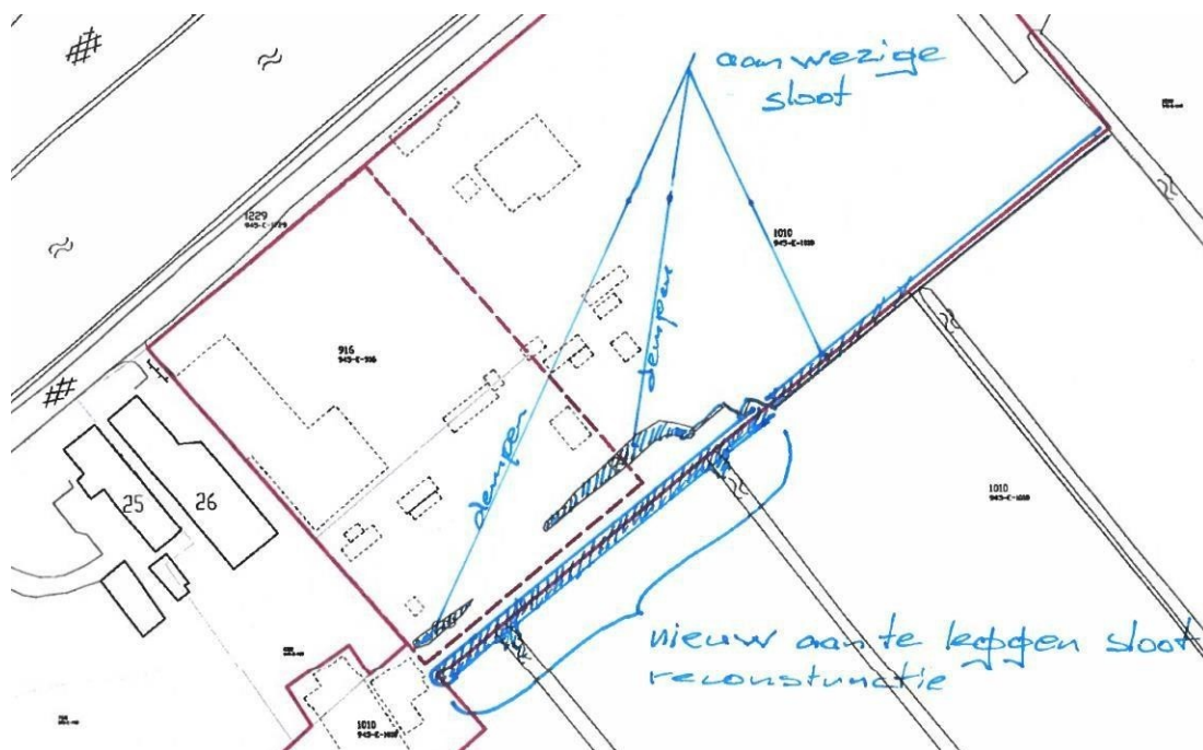
Fig. 3.6 Wijziging waterloop
